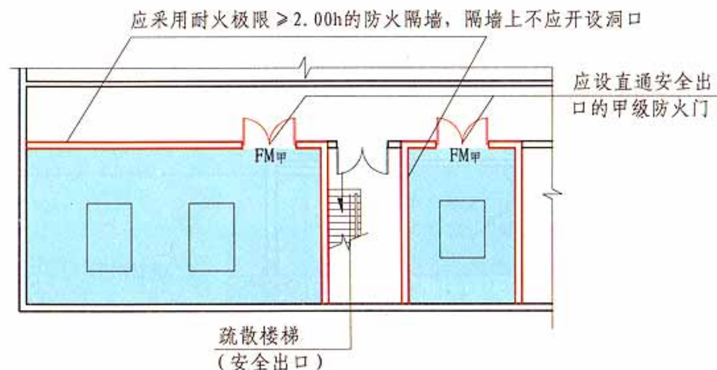
锅炉房、变压器室确需布置在民用建筑内地下层时 平面示意图
