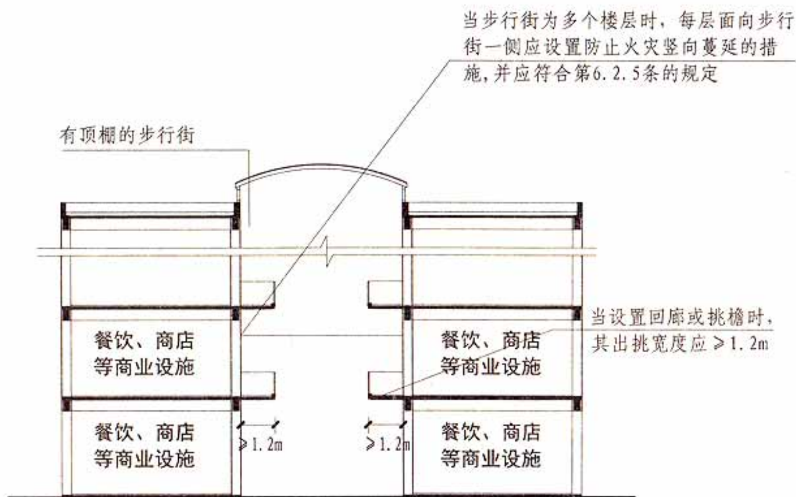
步行街两侧为多个楼层时剖面示意图
