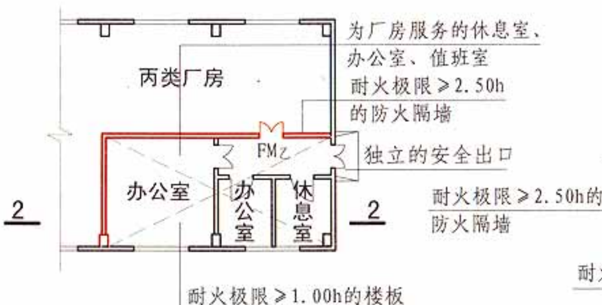
丙类厂房内设置办公室、休息室 平面示意图
