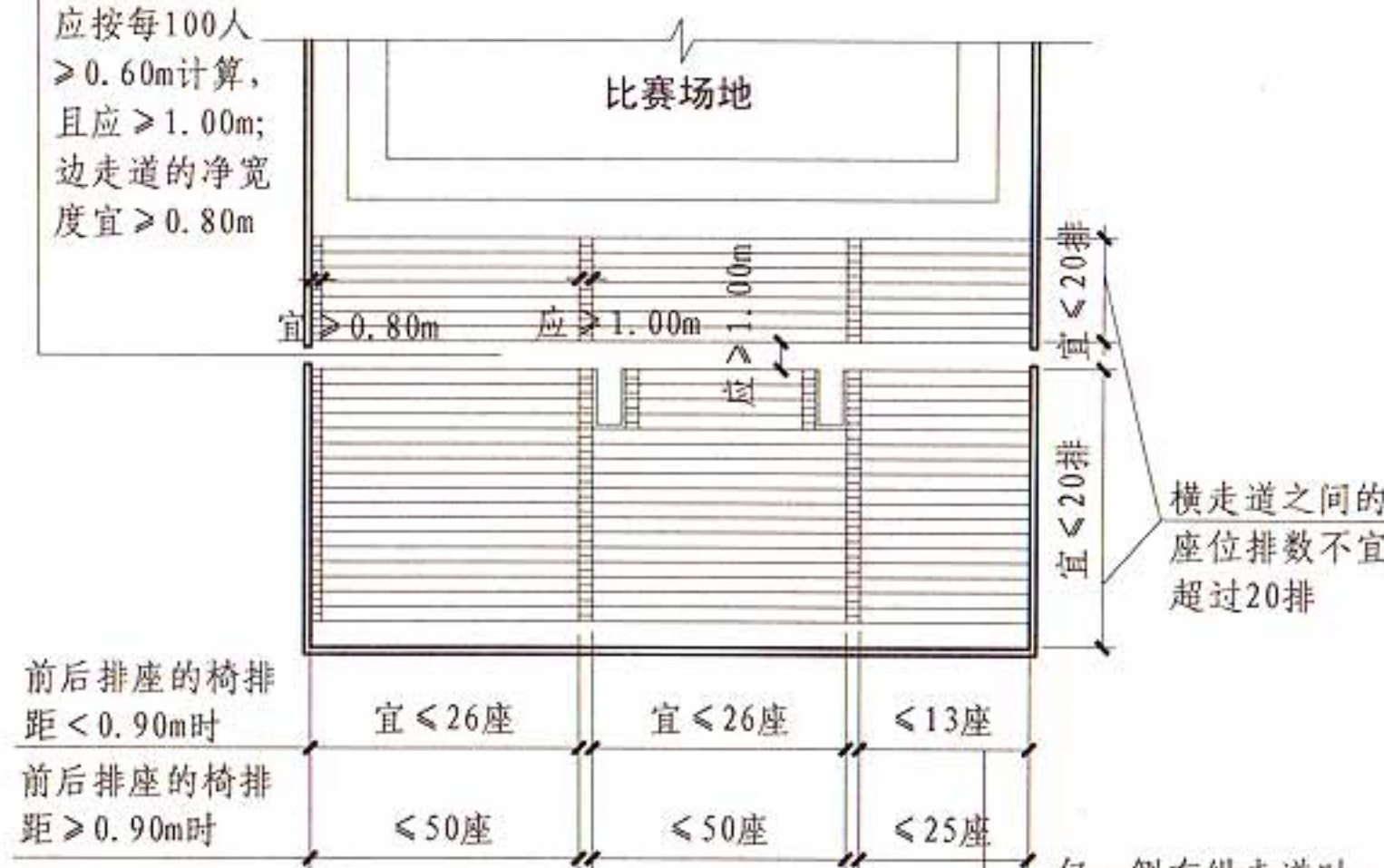
观众厅 (体育馆) 平面示意图
