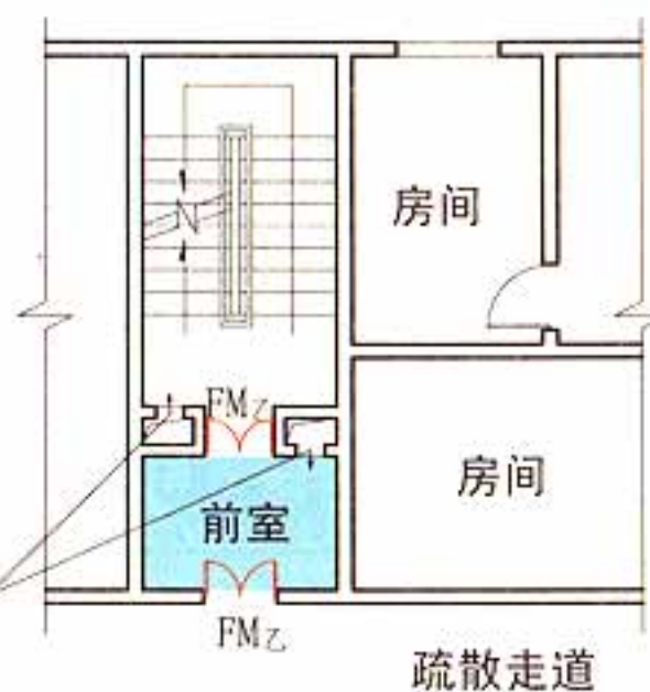
不能自然通风或自然通风不能满足要求的防烟楼梯间
