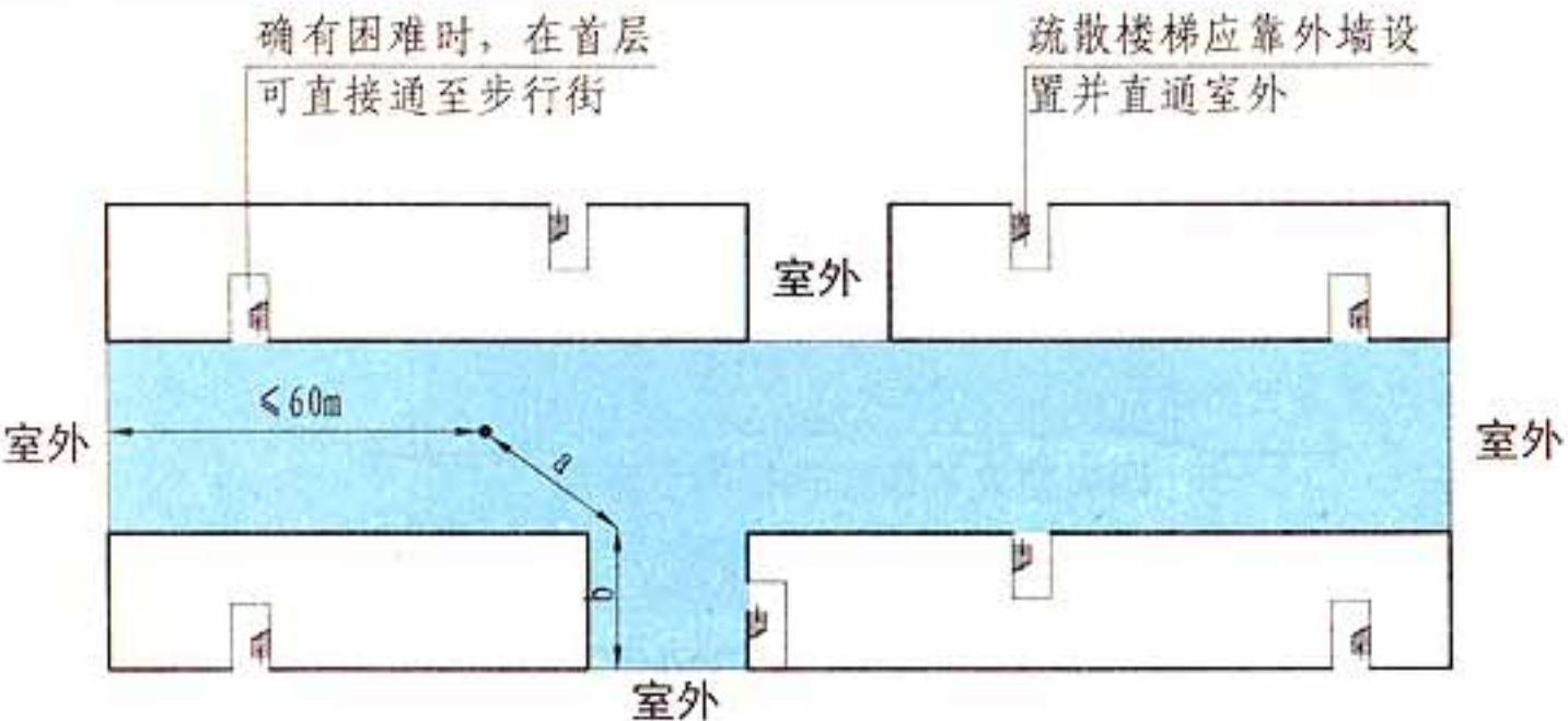
首层平面示意图 5.3.6 图示5
