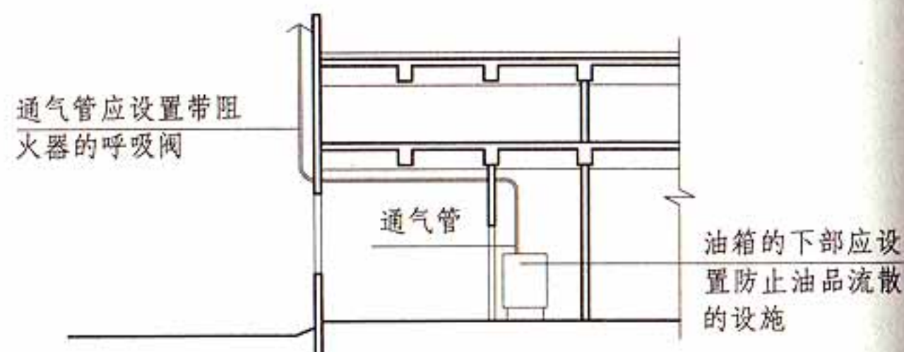
剖面示意图
