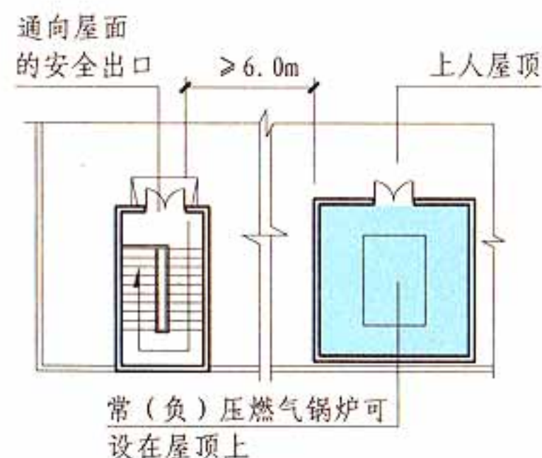
屋顶平面示意图
