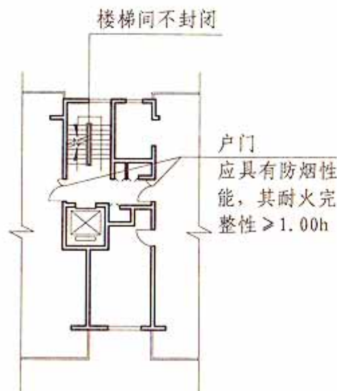
21m<建筑高度≤33m的住宅建筑
