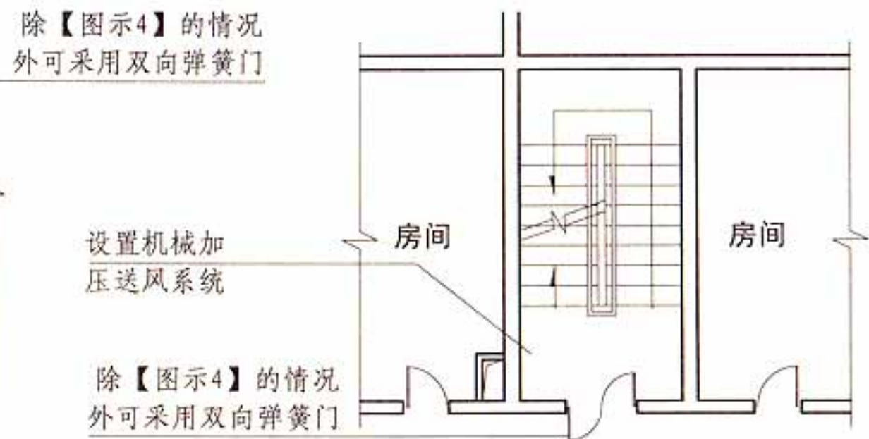
不能自然通风或自然通风不能满足要求的封闭楼梯间
