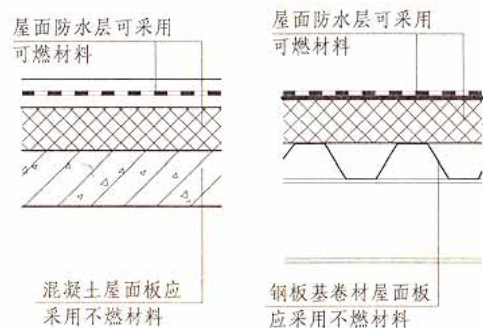
一、二级耐火等级厂房（仓库） 屋面板材料
