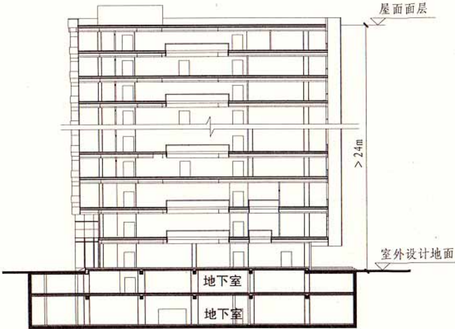
高层厂房、仓库和高层民用建筑 剖面示意图
