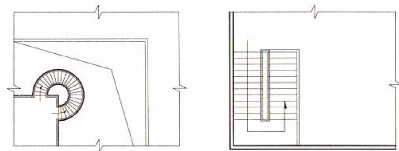
敞开楼梯 平面示意图
