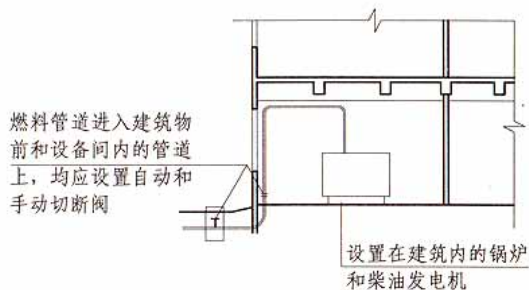
剖面示意图
