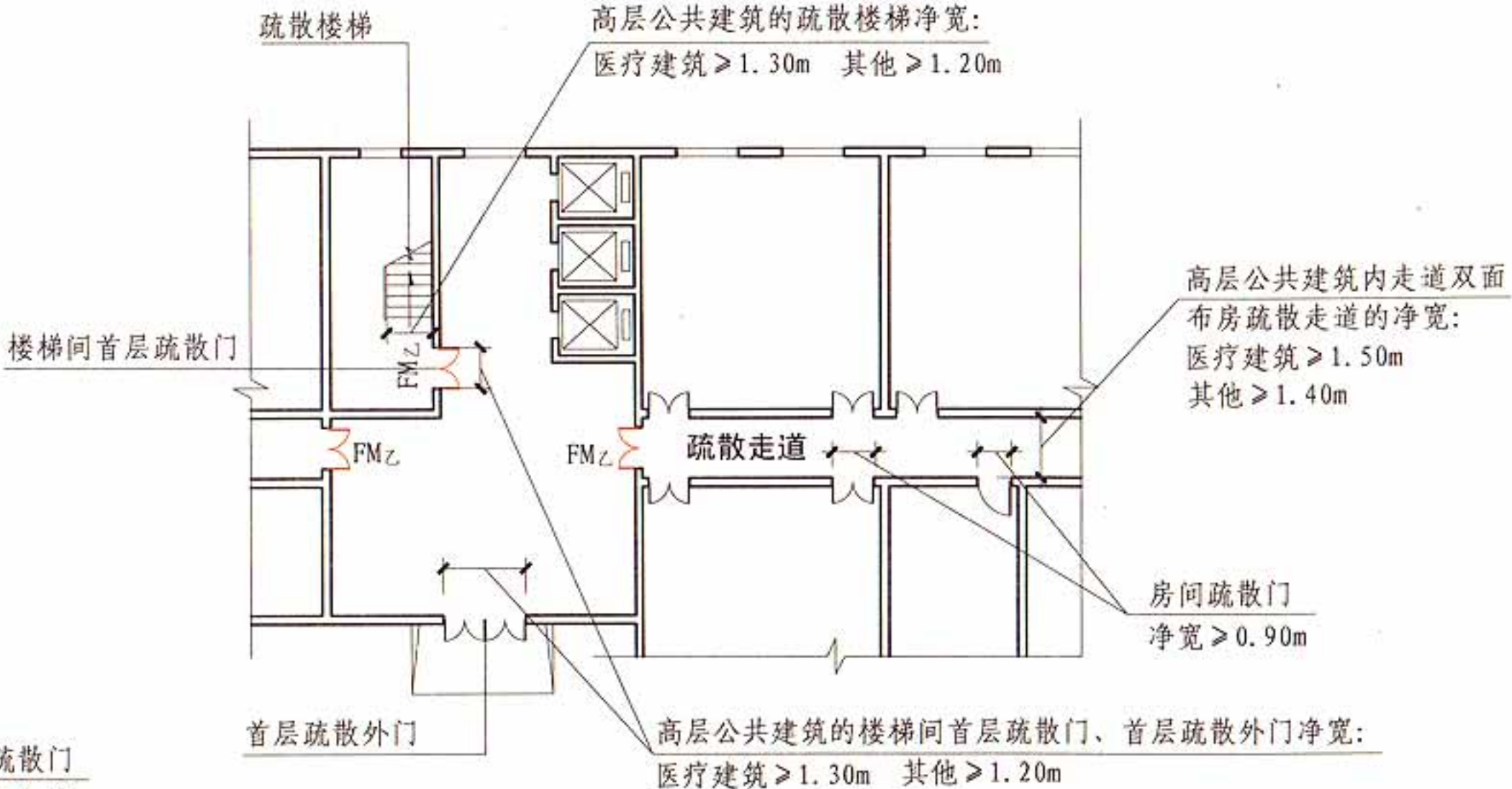
高层公共建筑 平面示意图
