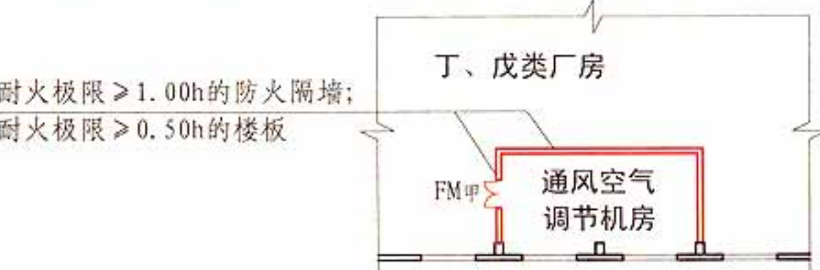
平面示意图
