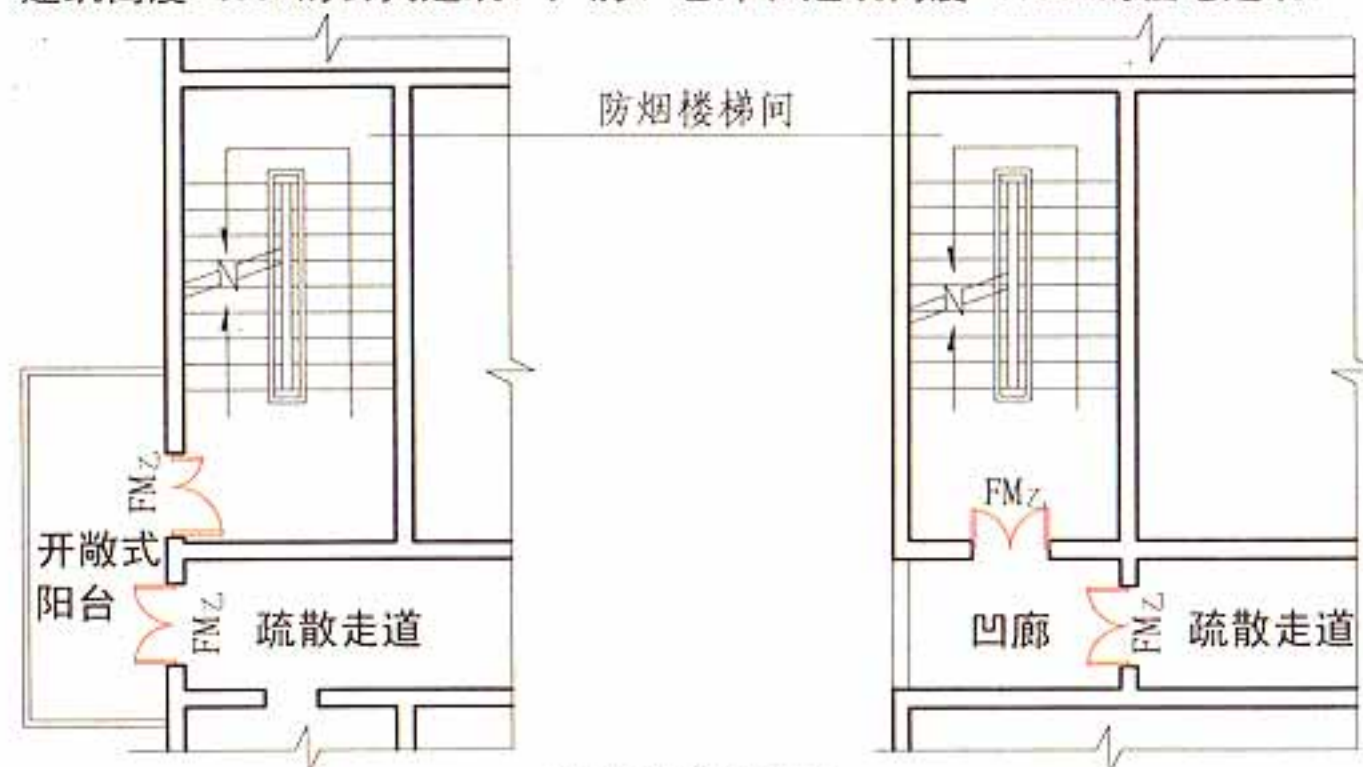
防烟楼梯间前室
