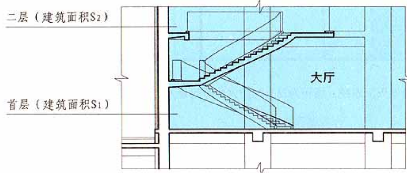
敞开楼梯 剖面示意图
