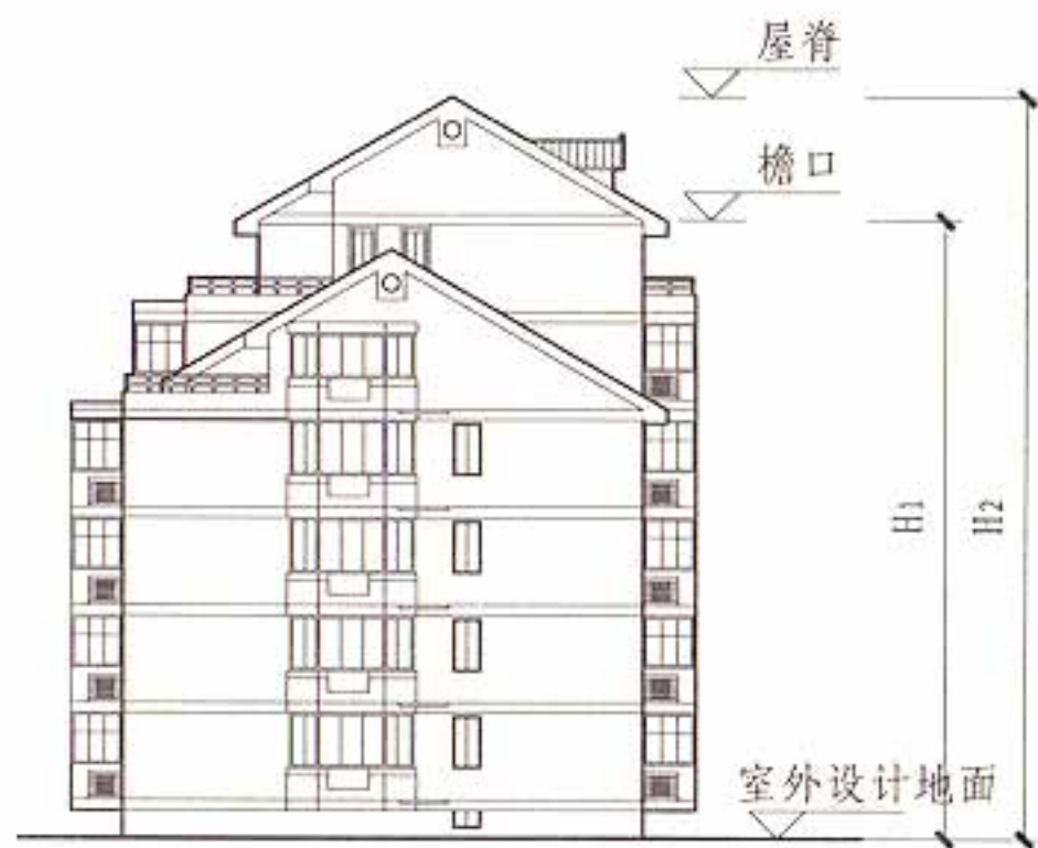
A.0.1 图示1 坡屋面建筑剖面示意图
