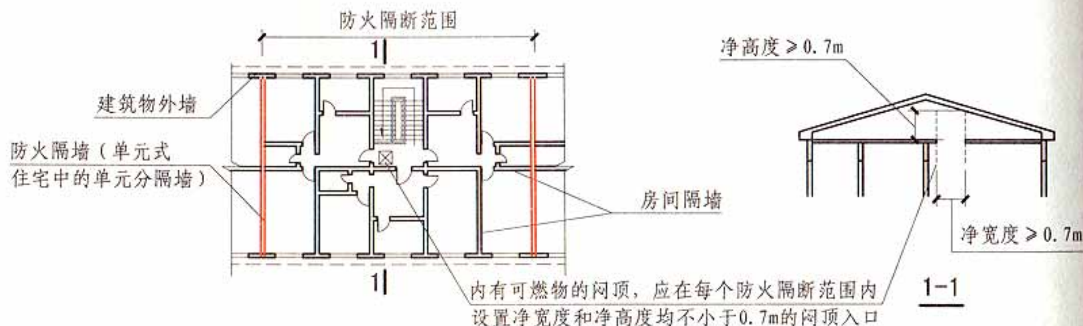
住宅顶层平面示意图
