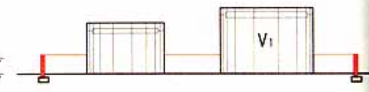
浮顶储罐组 V_0 \geq 0.5V_1 V_1 为最大储罐的容量 V_0 为防火堤内的有效容量
