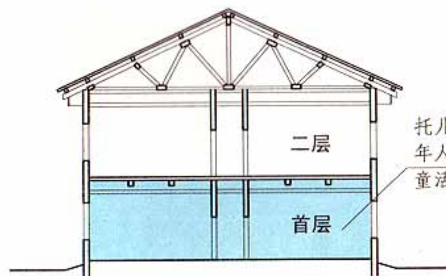
剖面示意图 四级耐火等级建筑
