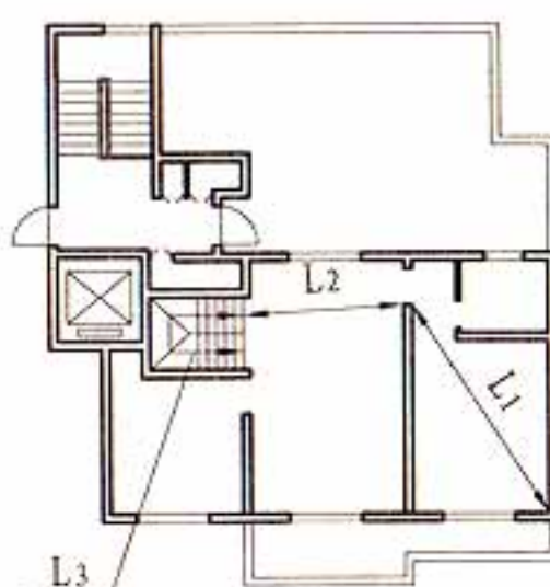
跃层平面
