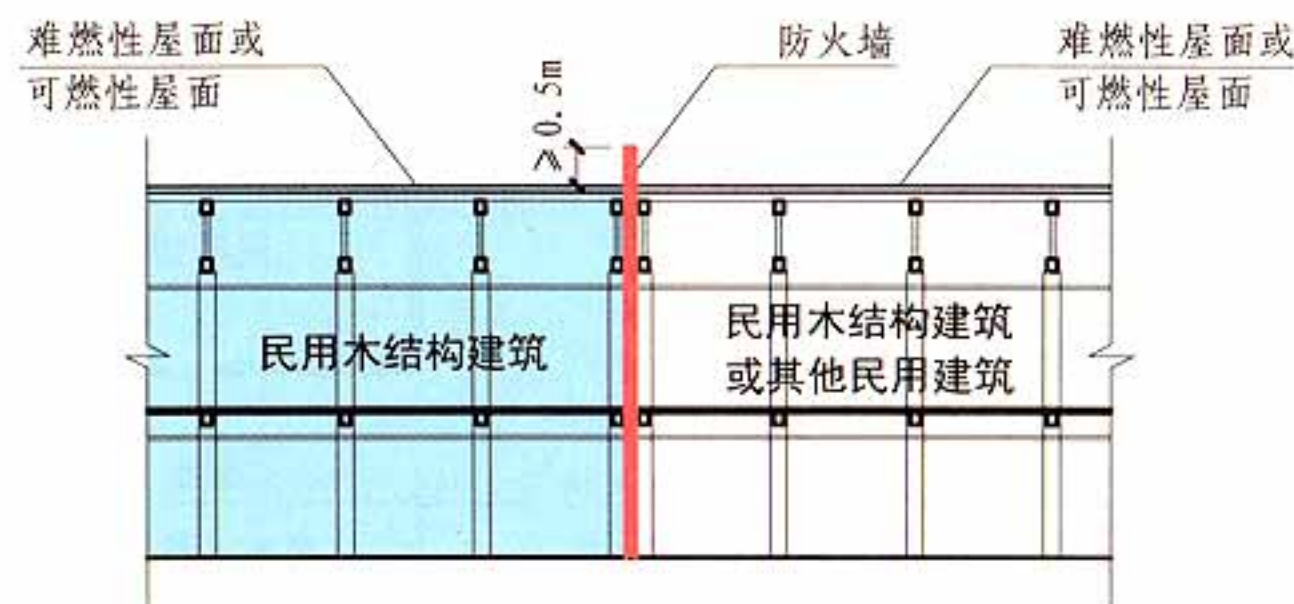
剖面示意图
