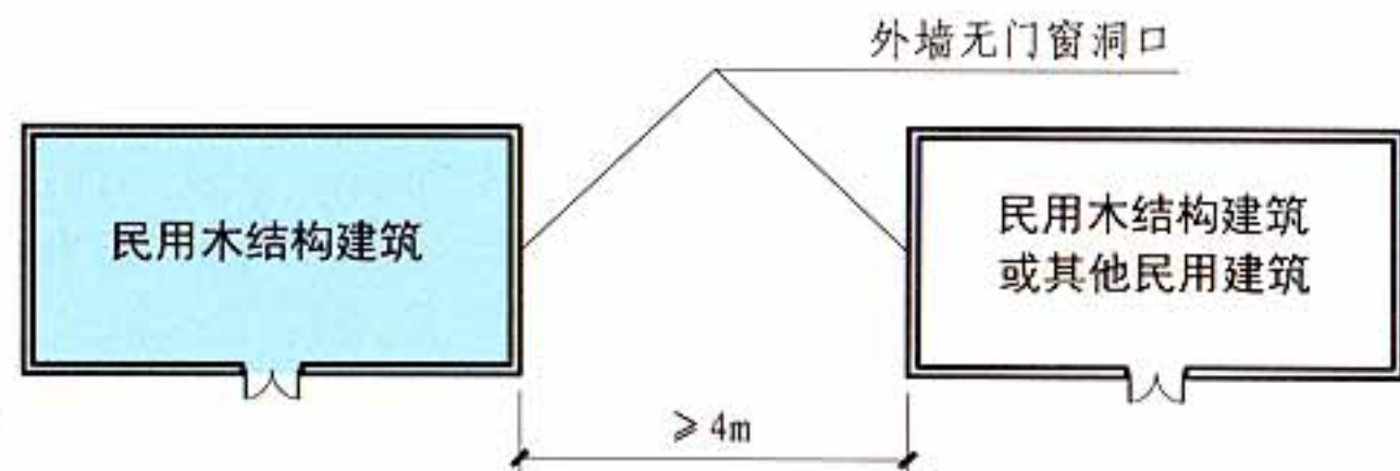
平面示意图 11.0.10 图示3
