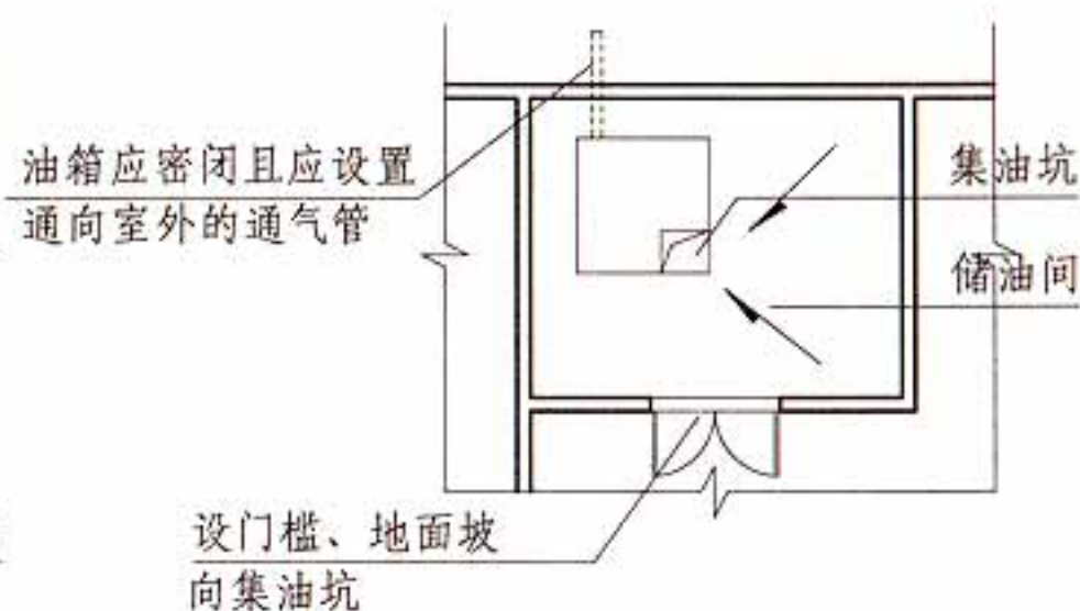
平面示意图
