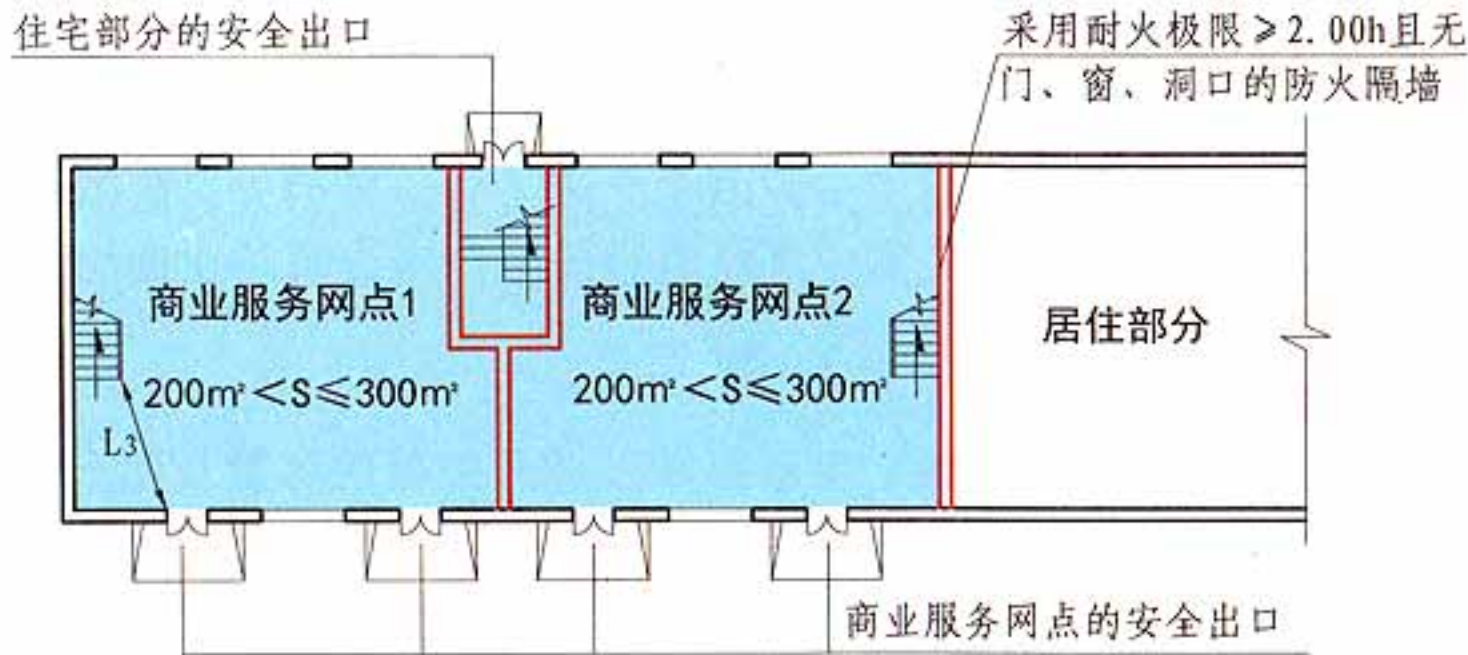
首层平面示意图
