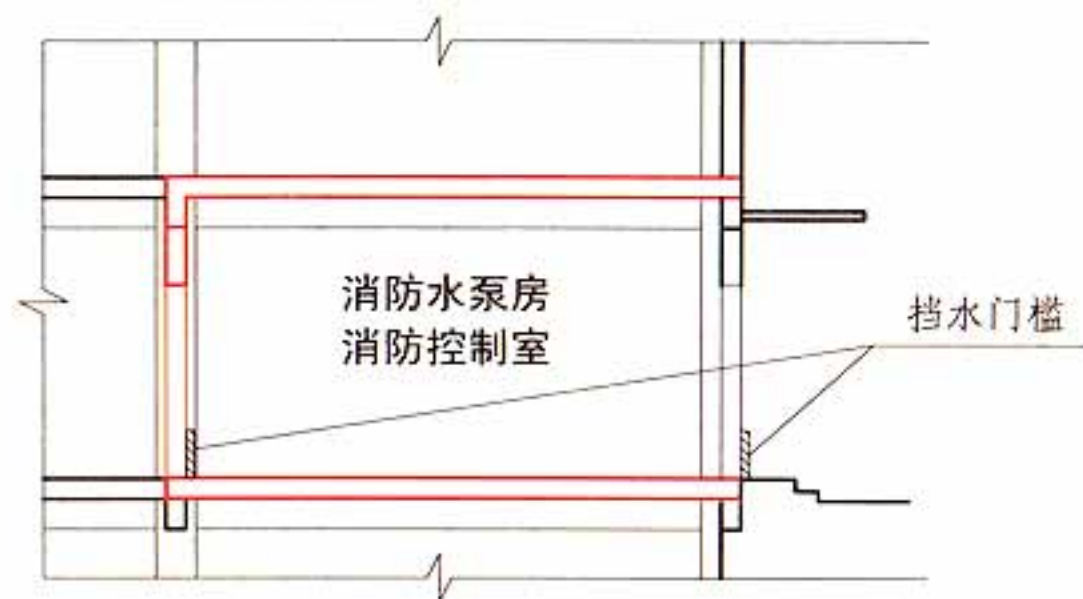
设在建筑首层的消防水泵房或消防控制室
