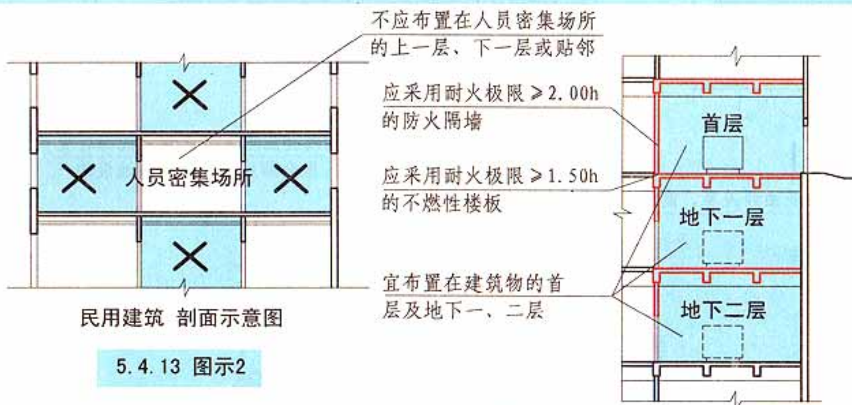
布置在民用建筑内的柴油发电机房 剖面示意图
