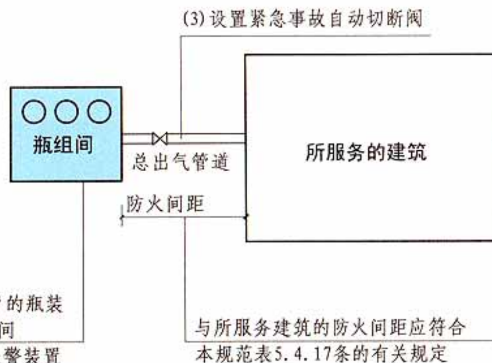
平面示意图
