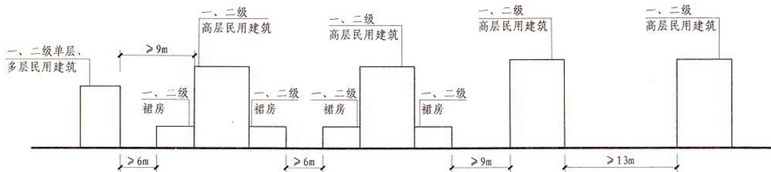
一、二级民用建筑之间的防火间距
