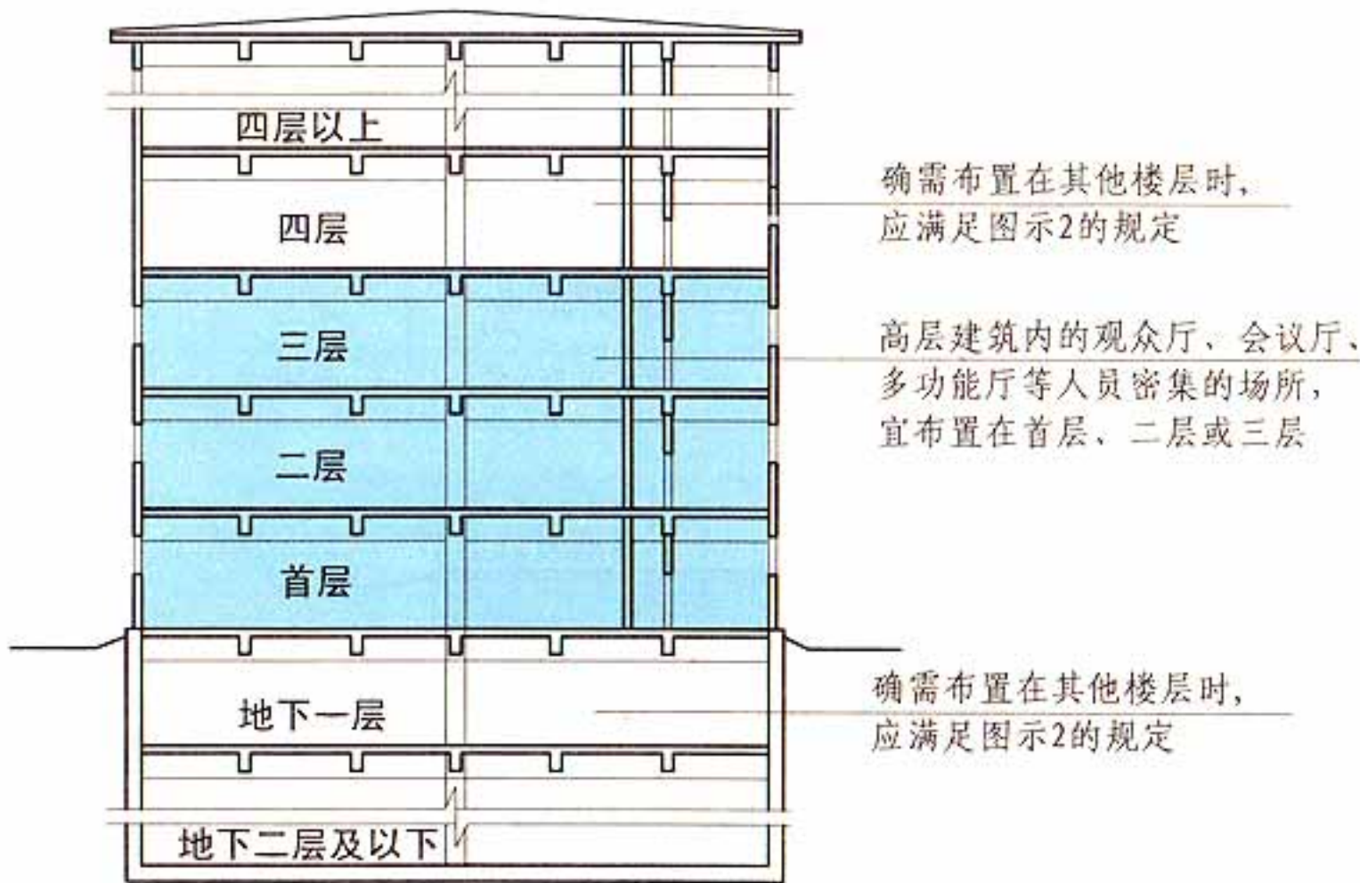
高层建筑剖面示意图
