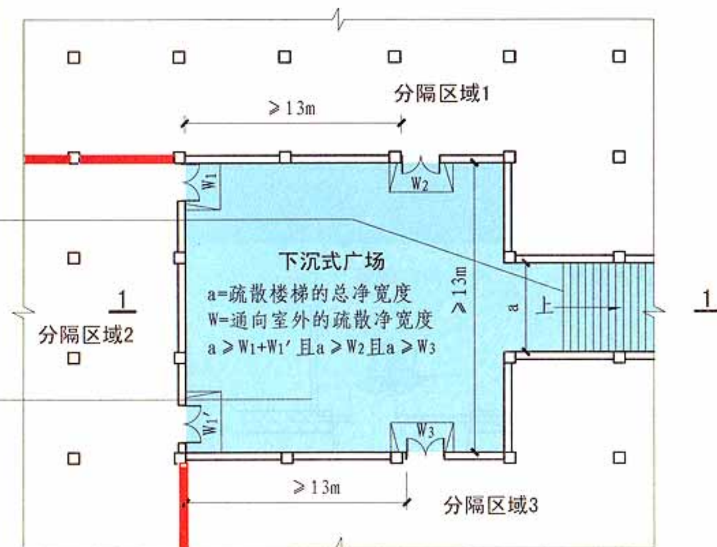
地下一层平面示意图
