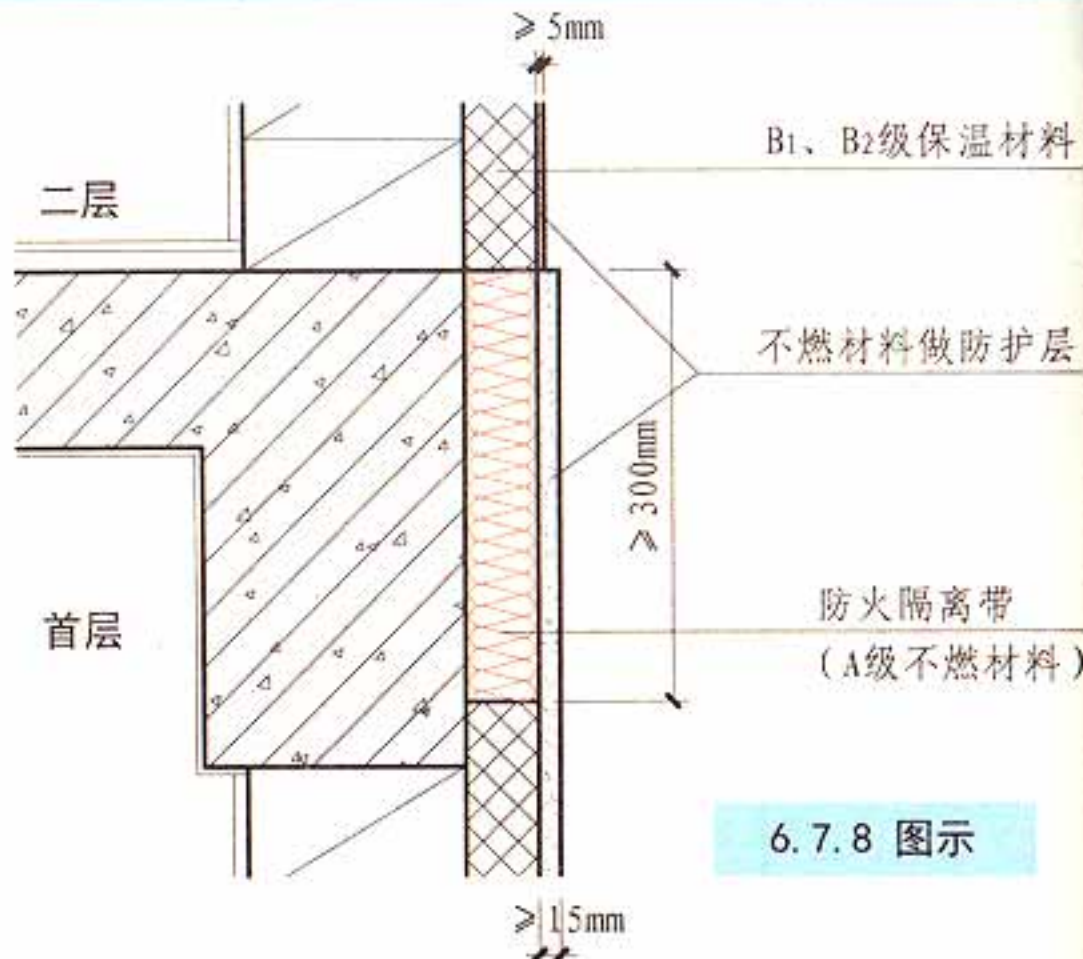
建筑高度与基层墙体、装饰层之间有空腔的建筑外墙保温系统的技术要求
