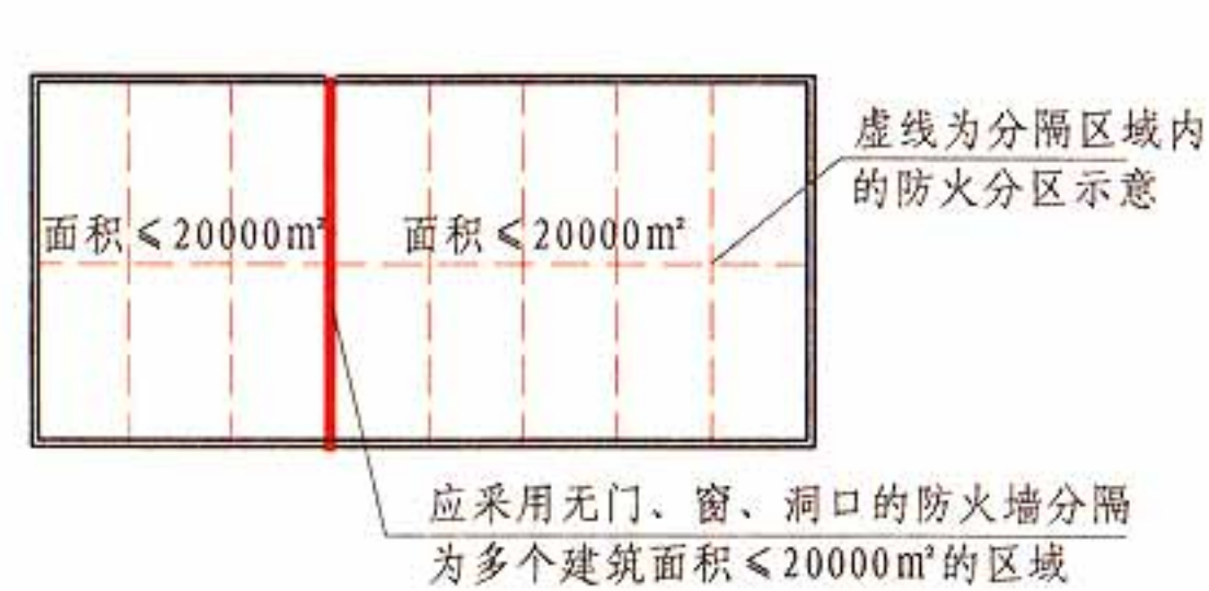
总建筑面积>20000m 2 的地下或半地下商店 平面示意图
