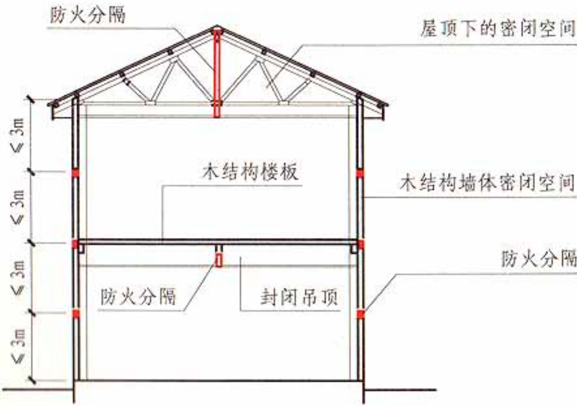
木结构建筑 剖面示意图
