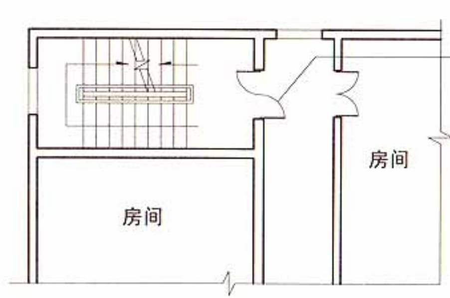
能自然通风且自然通风能满足要求的封闭楼梯间
