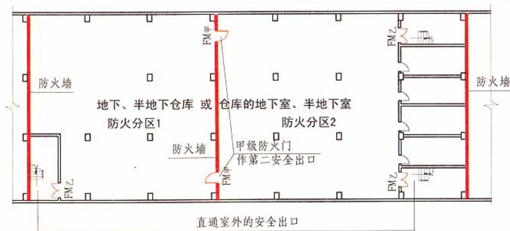
平面示意图
