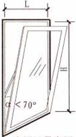
内开下悬窗开 窗角度小于70°
