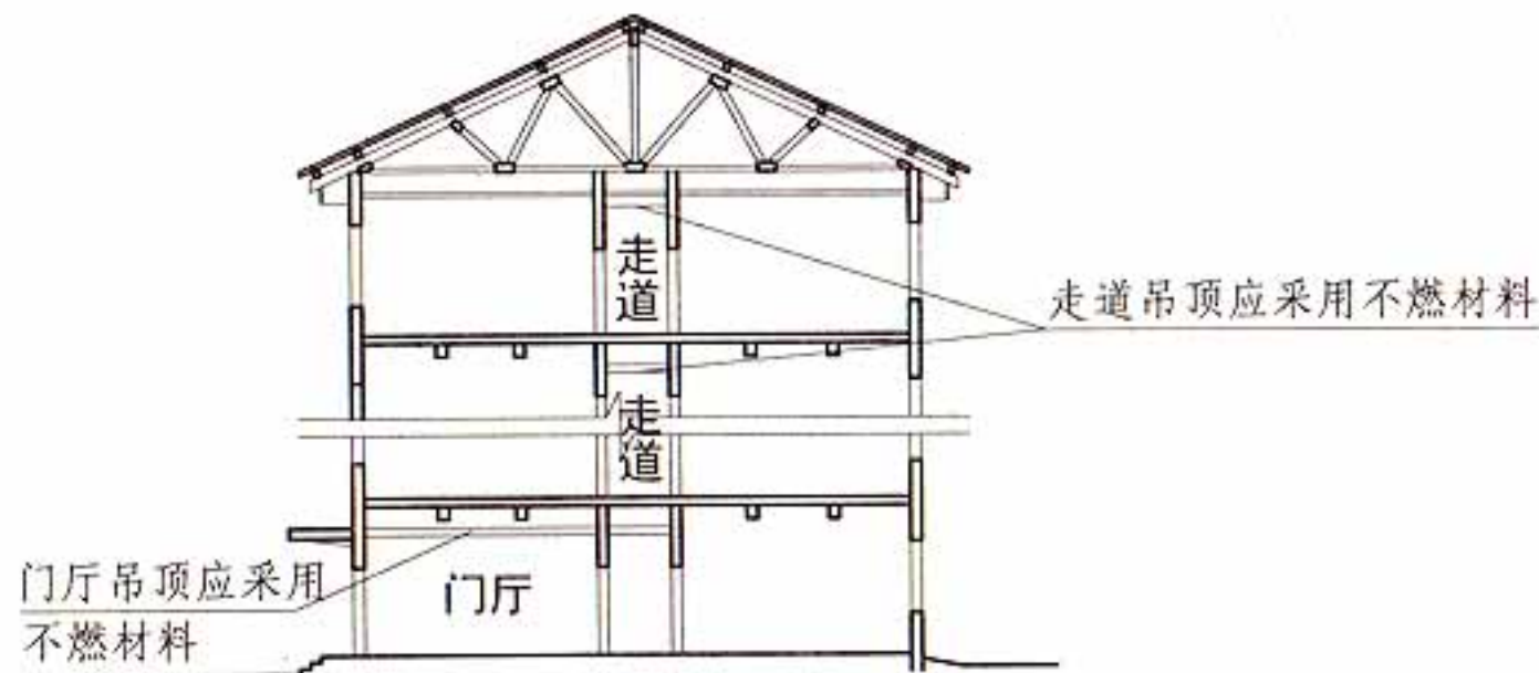
二、三级耐火等级建筑门厅、走道的吊顶 5.1.7 图示2
