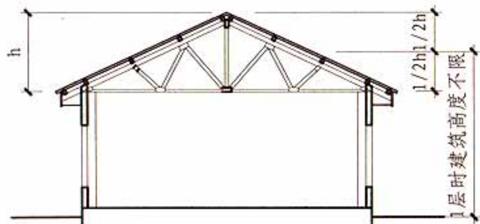
胶合木结构建筑
