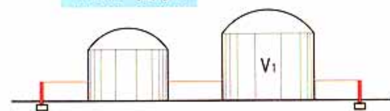
固定顶储罐组（地上式） V_0 \geq V_1 V_1 为最大储罐的容量 V_0 为防火堤内的有效容量
