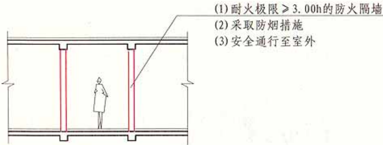
避难走道剖面示意图
