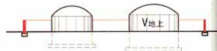
固定顶储罐组（半地下式） V_0 \geq V_{\text{地上}} V_{\text{地上}} 为最大储罐高出地面的容量 V_0 为防火堤内的有效容量
