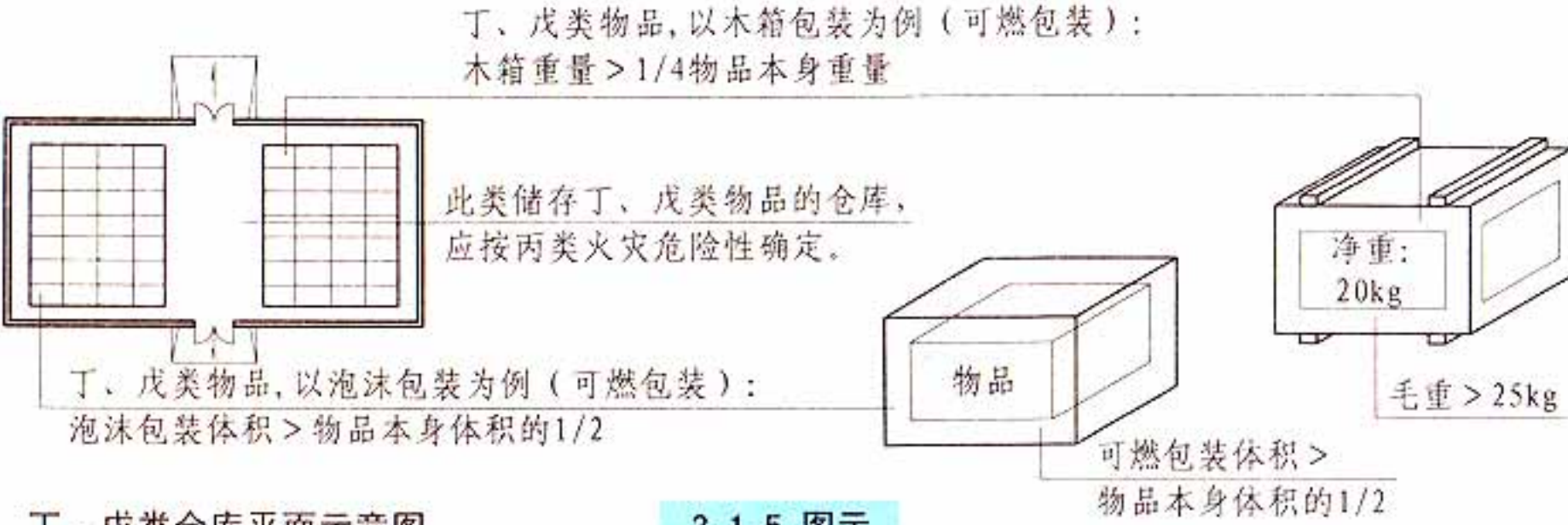
丁、戊类仓库平面示意图
