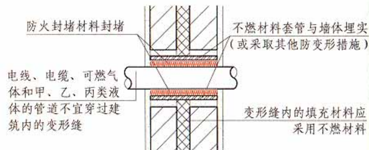
剖面示意图
