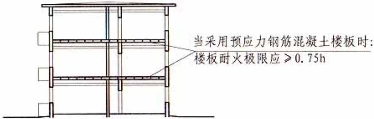
二级耐火等级的多层住宅建筑 5.1.6 图示2
