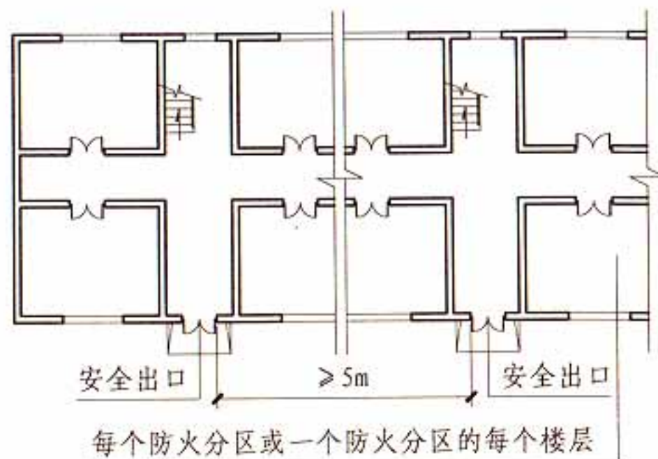
首层平面示意图
