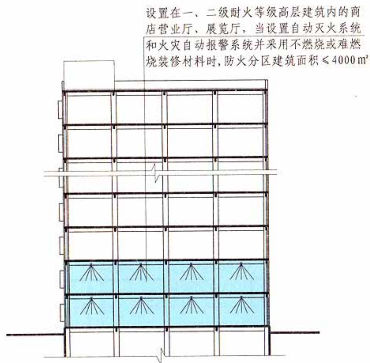
一、二级耐火等级高层建筑剖面示意图
