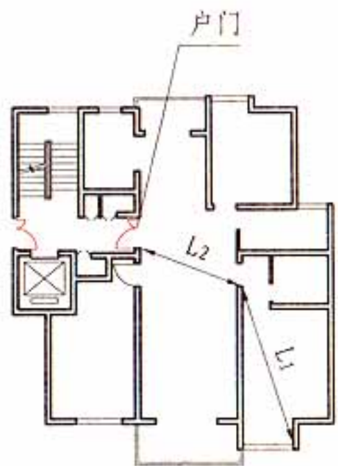
住宅建筑户内任一点至直通疏散走道的户门的直线距离
