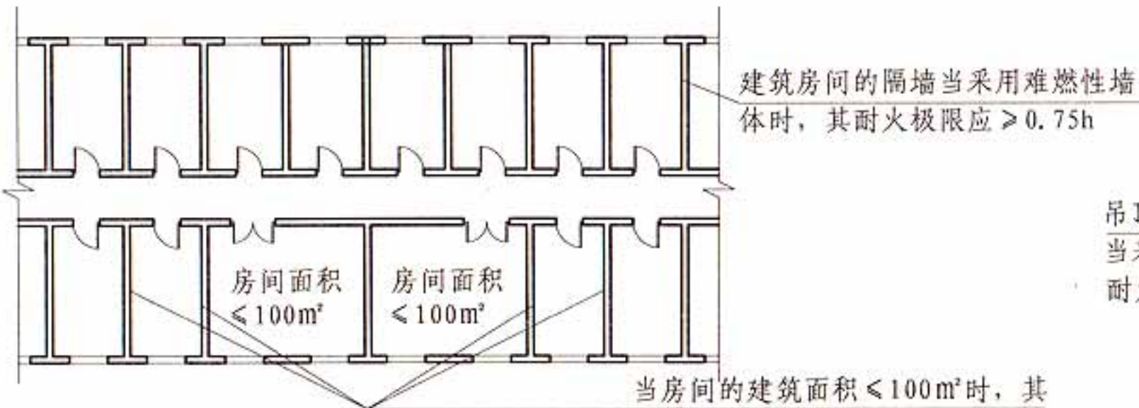
二级耐火等级建筑的房间隔墙 5.1.6 图示1
