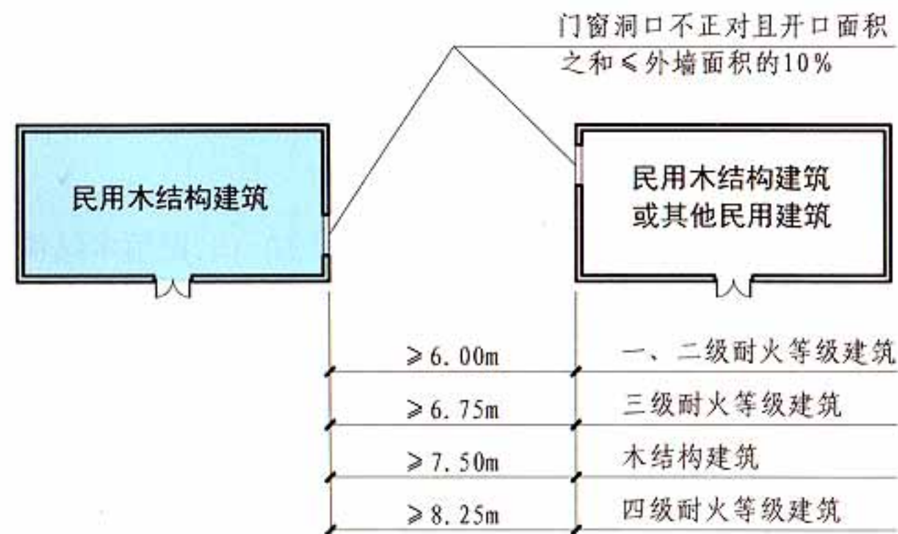
平面示意图
