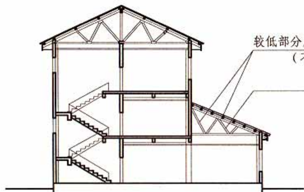
剖面示意图
