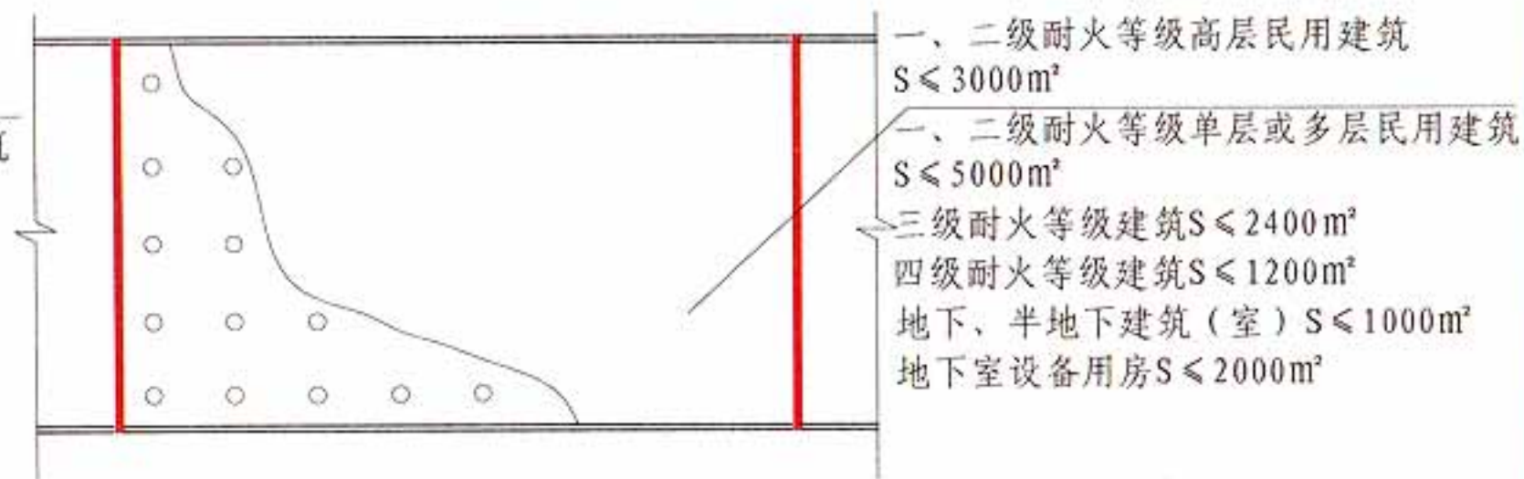
当建筑内设置自动灭火系统时防火分区的最大允许建筑面积S
