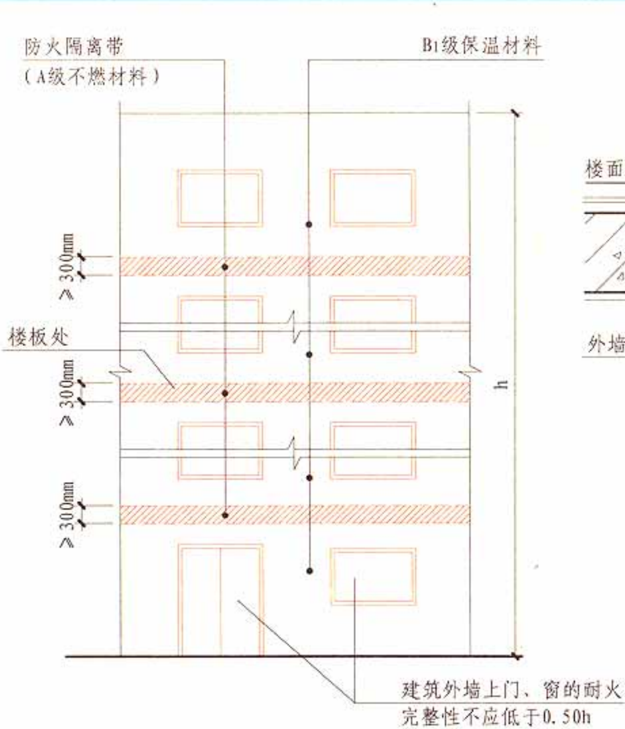
当采用B1级保温材料时，公共建筑建筑高度 h > 24\text{m} ；住宅建筑建筑高度 h > 27\text{m} 立面示意图
