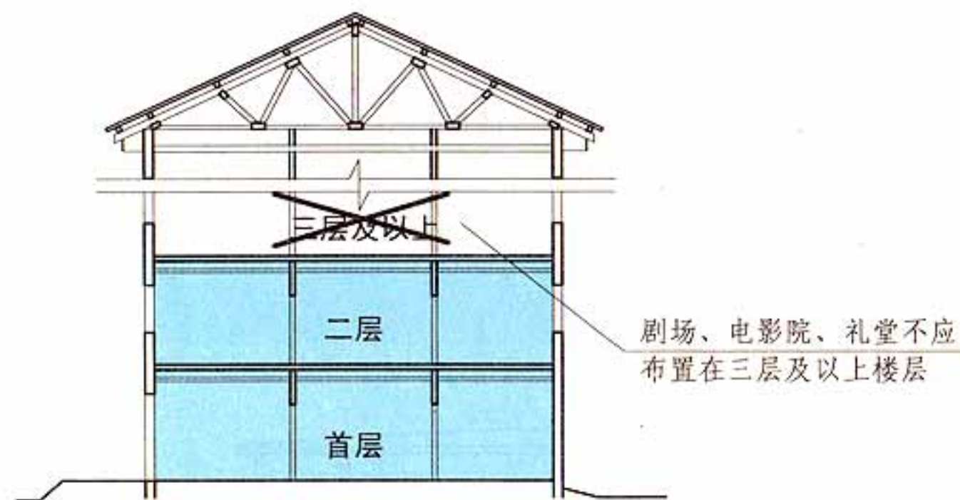
三级耐火等级建筑剖面示意图
