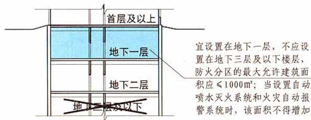
剖面示意图
