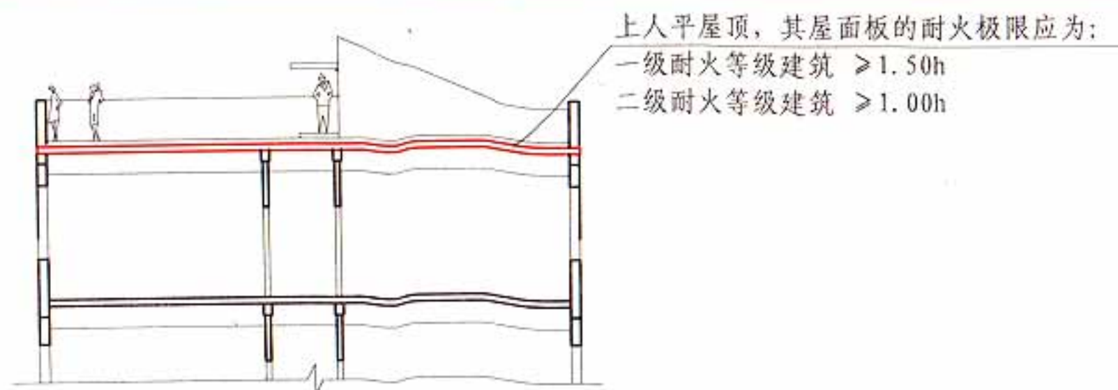
上人平屋顶剖面示意图 一、二级耐火等级建筑
