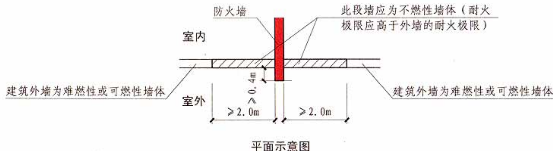
外墙为难燃性或可燃性墙体时，防火墙凸出墙外表面的规定
