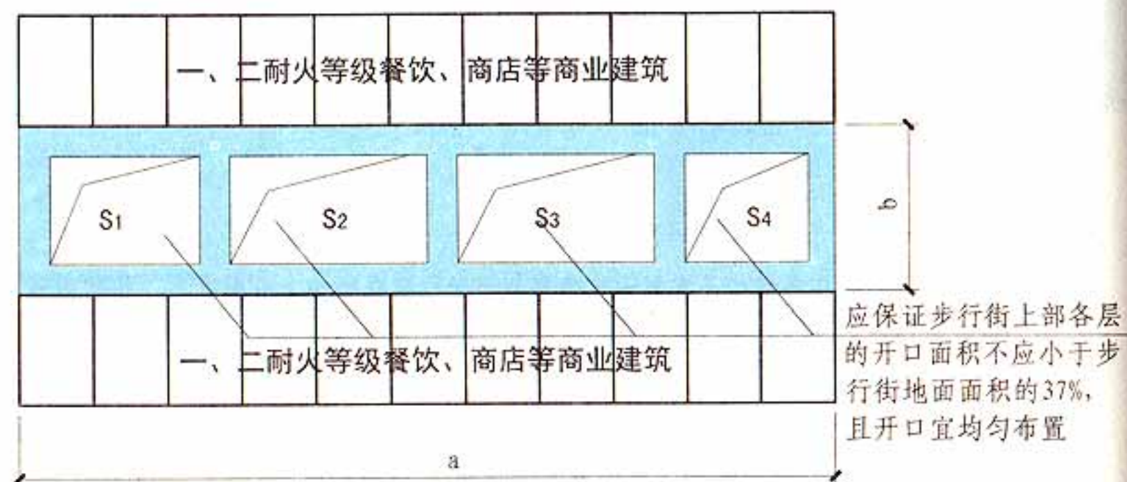
步行街两侧商铺在上部各层需设回廊或连接天桥时平面示意图
