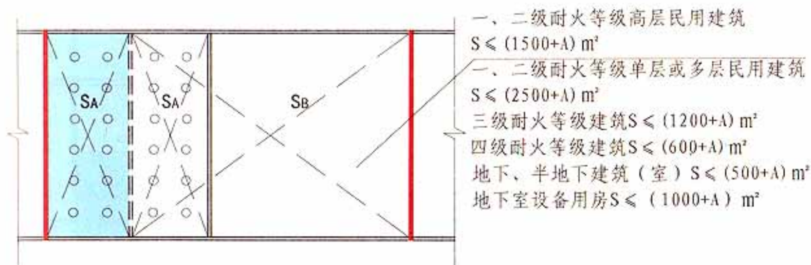
局部设置自动灭火系统(面积为2A)时防火分区的最大允许建筑面积S
