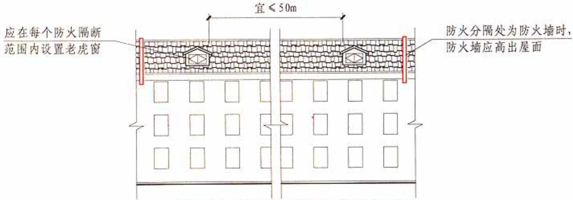
层数超过2层的三级耐火等级建筑内的闷顶
