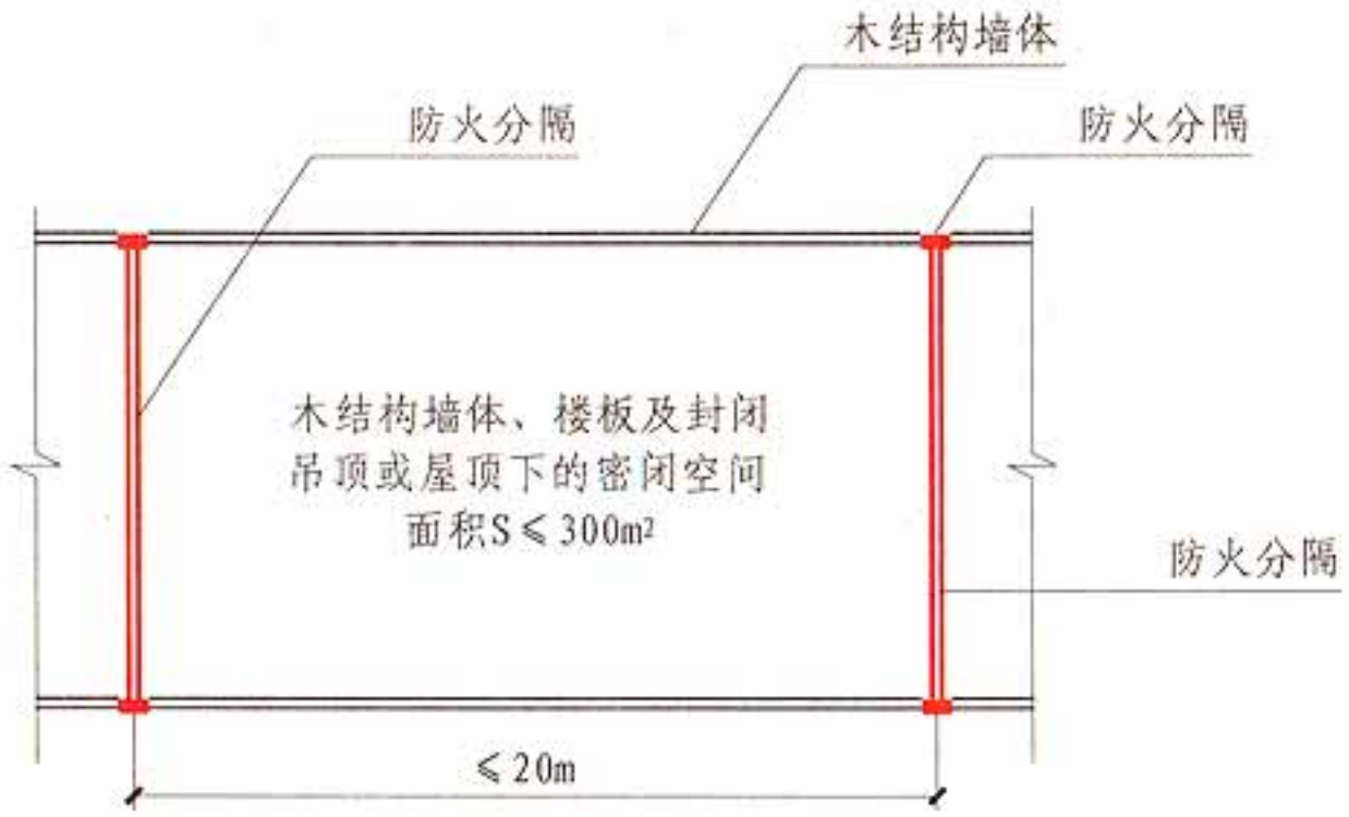
平面示意图
