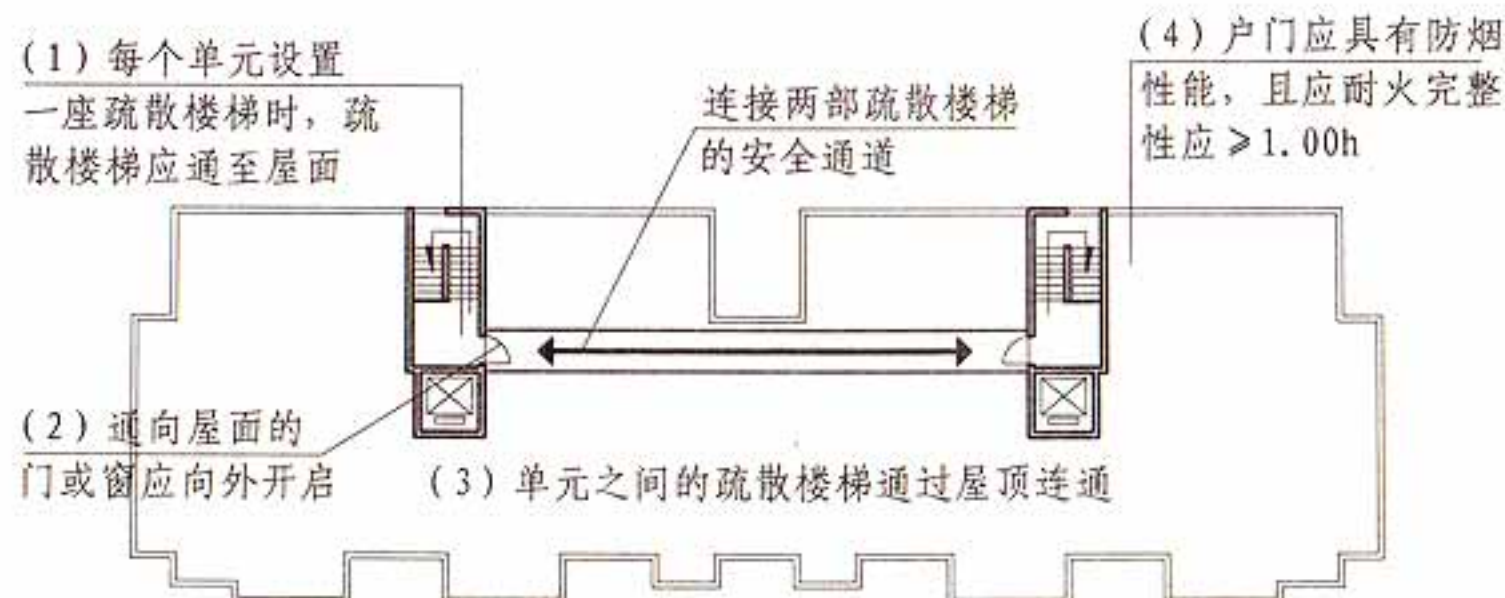
27m<建筑高度≤54m的住宅建筑 屋顶平面示意图
