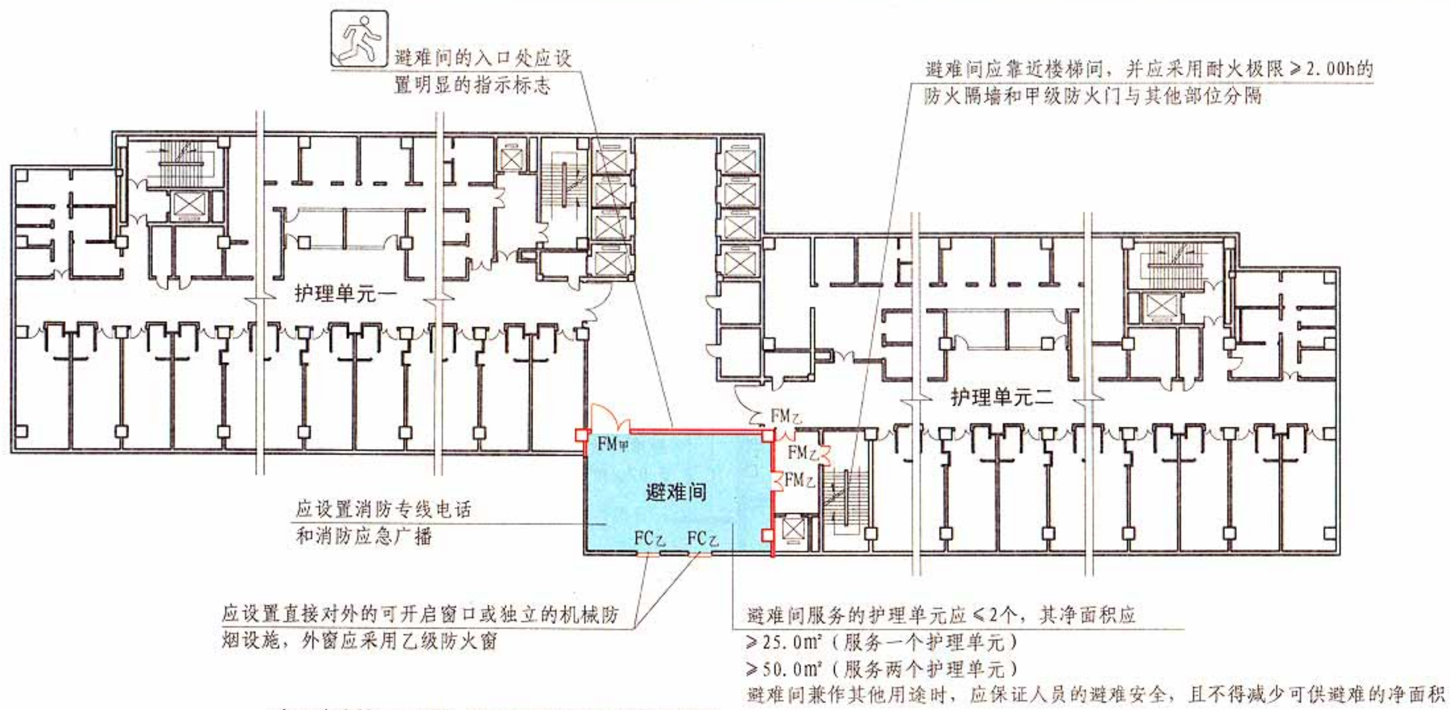
高层病房楼二层及以上的病房楼层和洁净手术部 避难间设置要求 平面示意图
