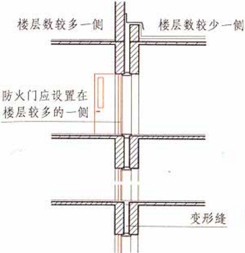
剖面示意图
