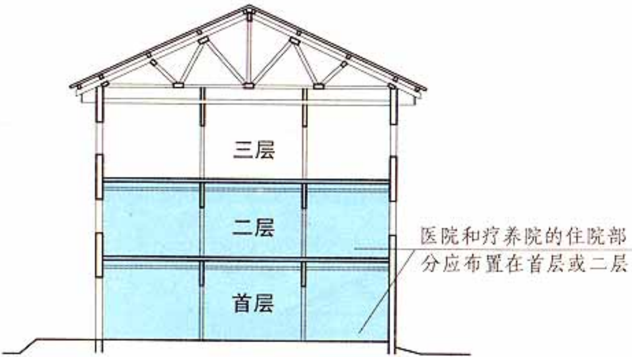
剖面示意图 三级耐火等级建筑 5.4.5 图示2
