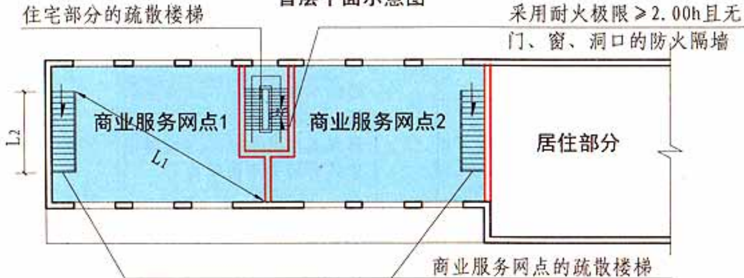
二层平面示意图
