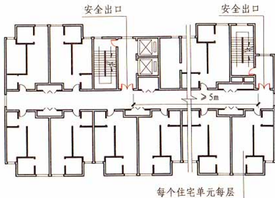
住宅单元标准层平面示意图
