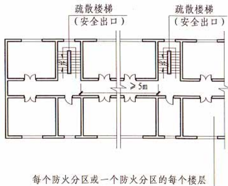
标准层平面示意图
