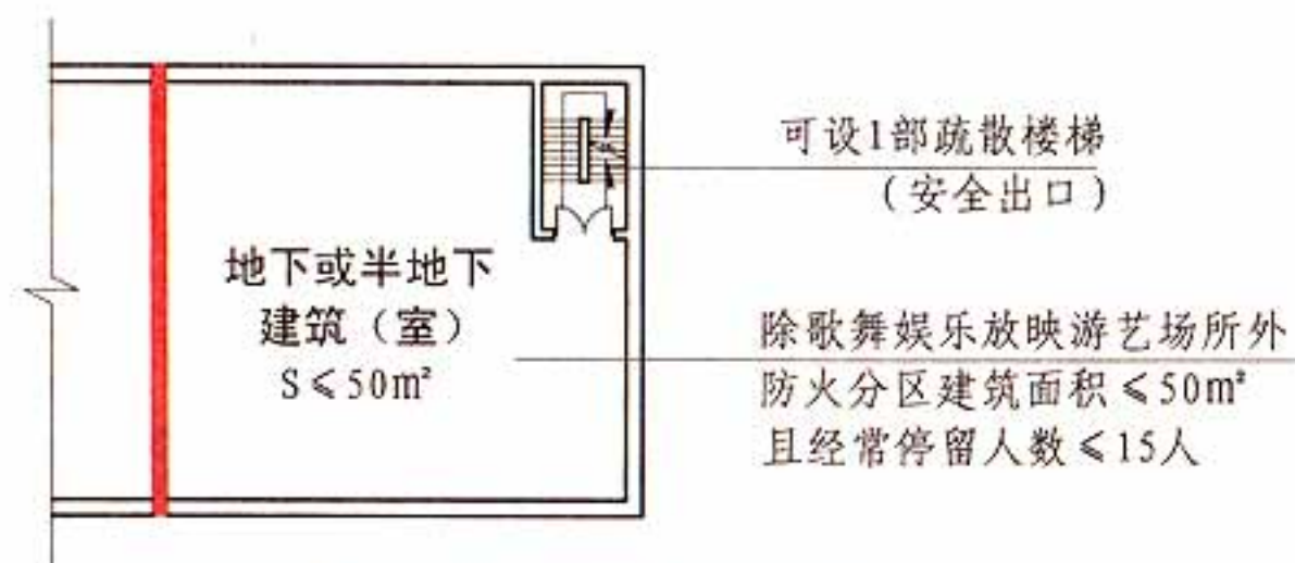
地下或半地下建筑(室)平面示意图
