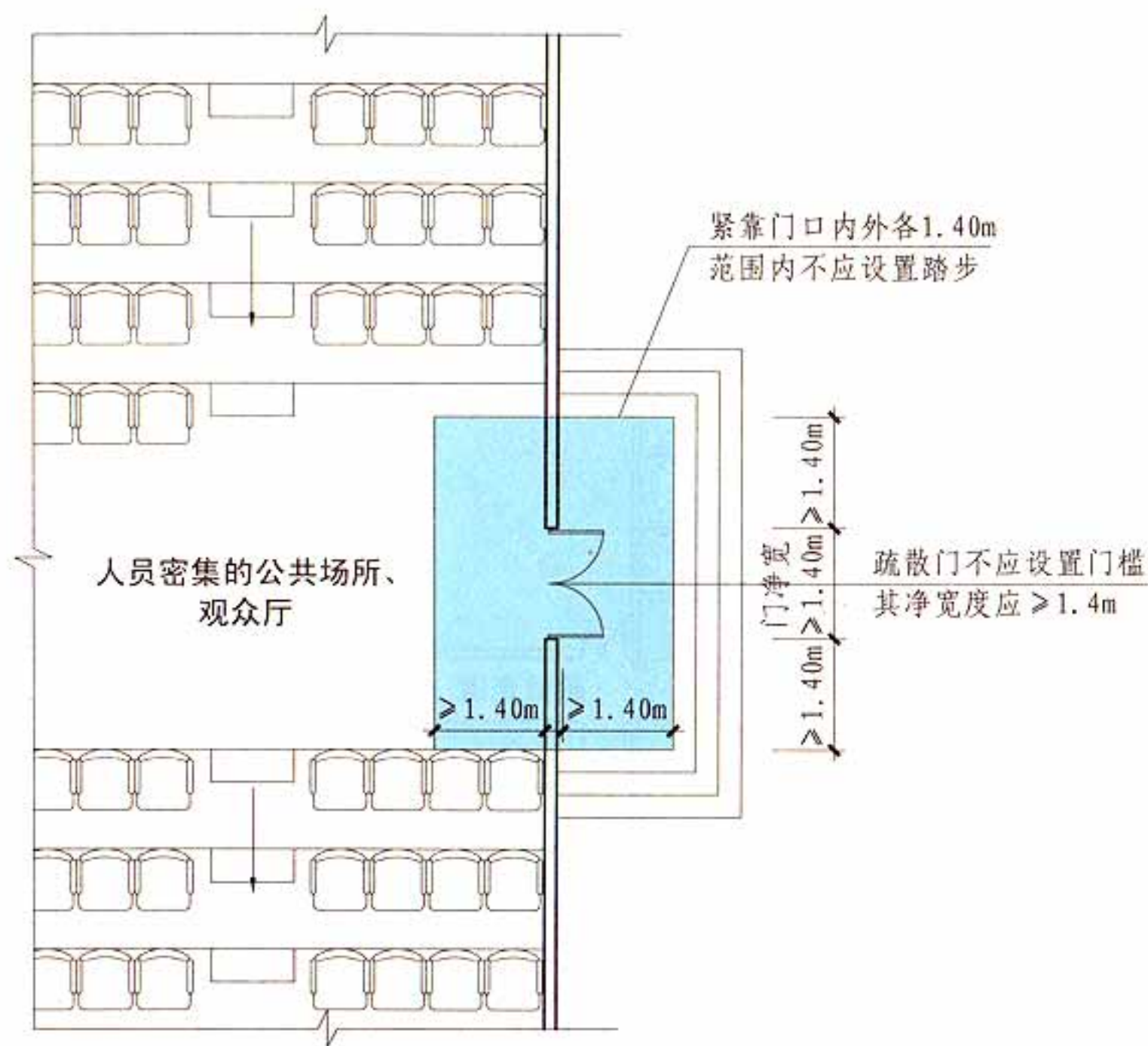
平面示意图
