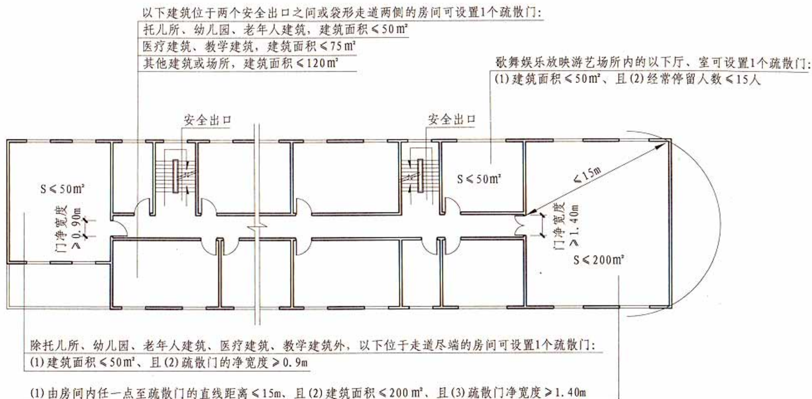
公共建筑 平面示意图
