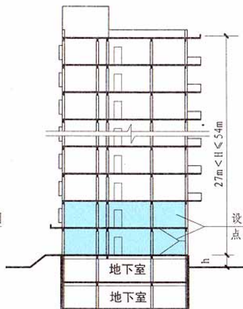
27\text{m} < \text{建筑高度} \leq 54\text{m} 的二类高层住宅建筑 (包括设置商业服务网点的住宅建筑)
