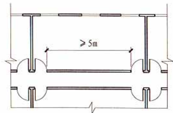
房间平面示意图
