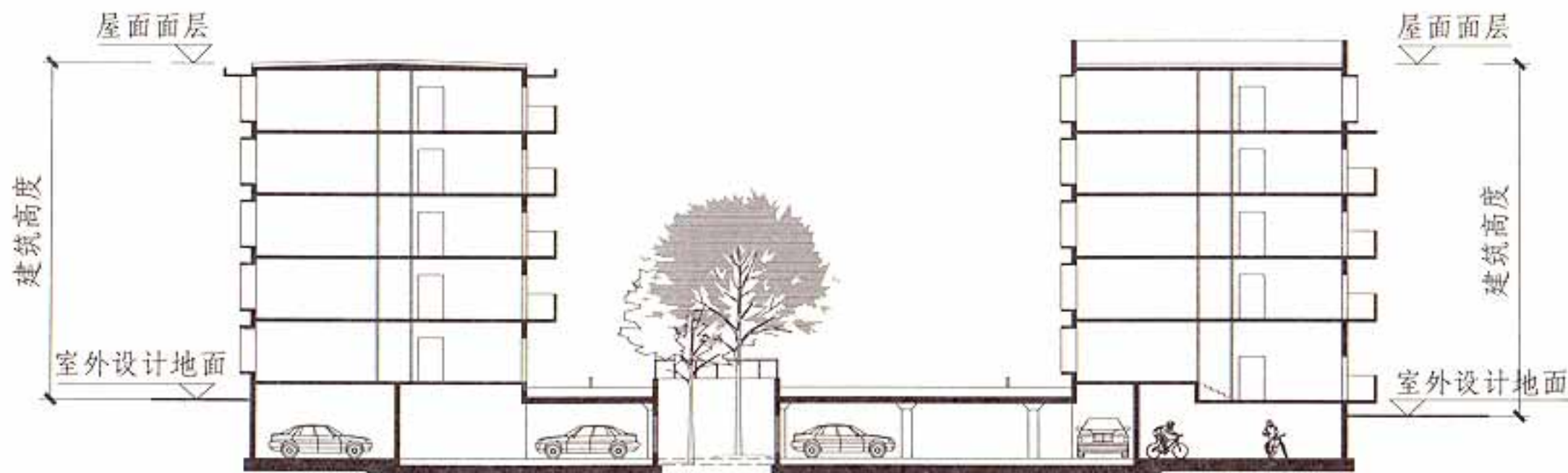
平屋面建筑剖面示意图
