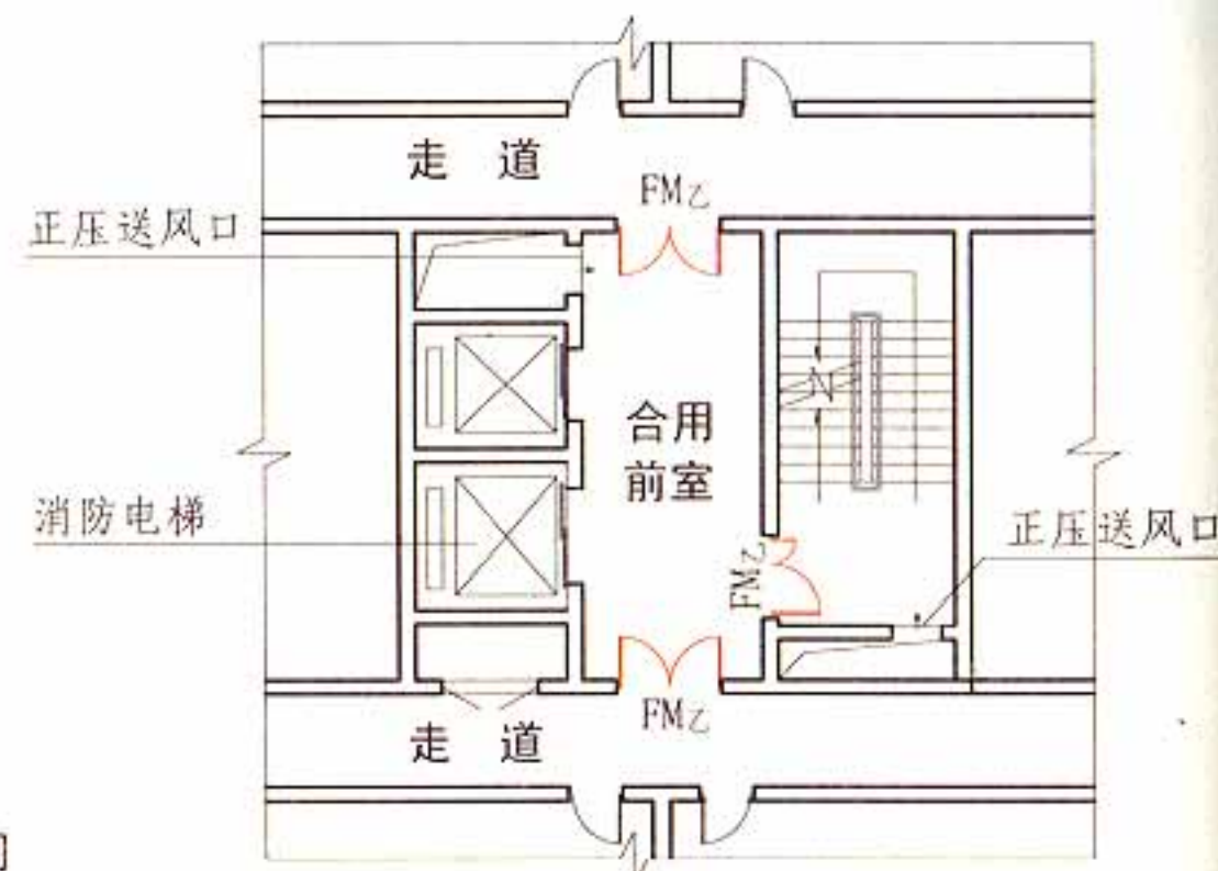
前室与消防电梯间前室合用的防烟楼梯间
