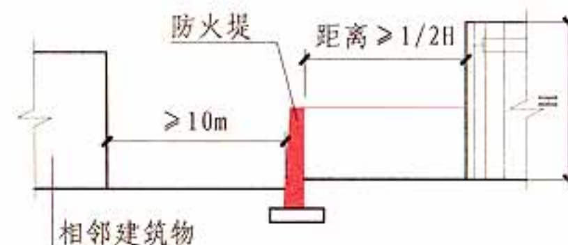
立面示意图 4.2.1 图示2
