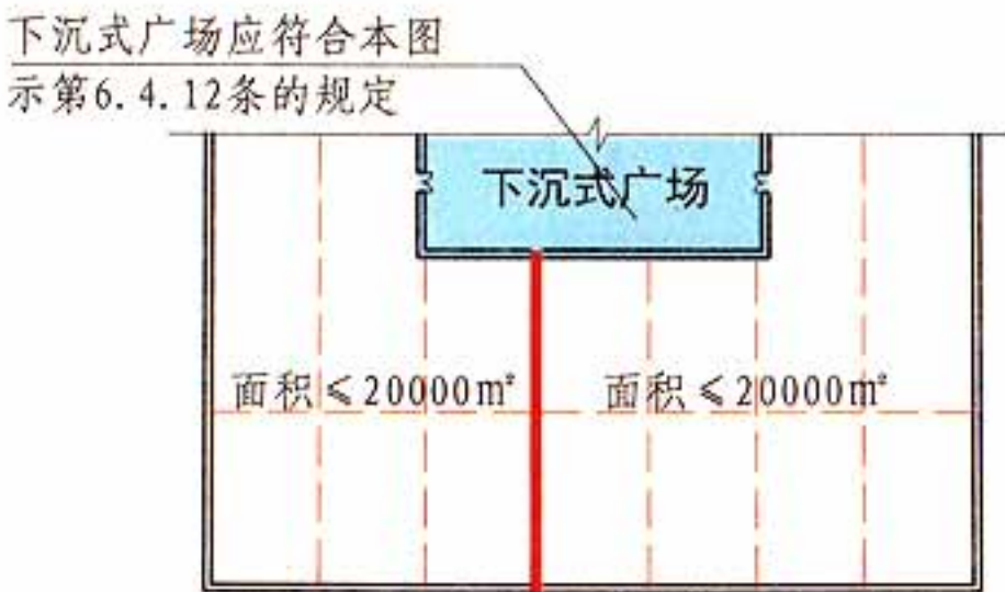
用下沉式广场方式连通 平面示意图
