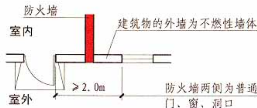
外墙为不燃性墙体时，防火墙不凸出墙外表面的规定
