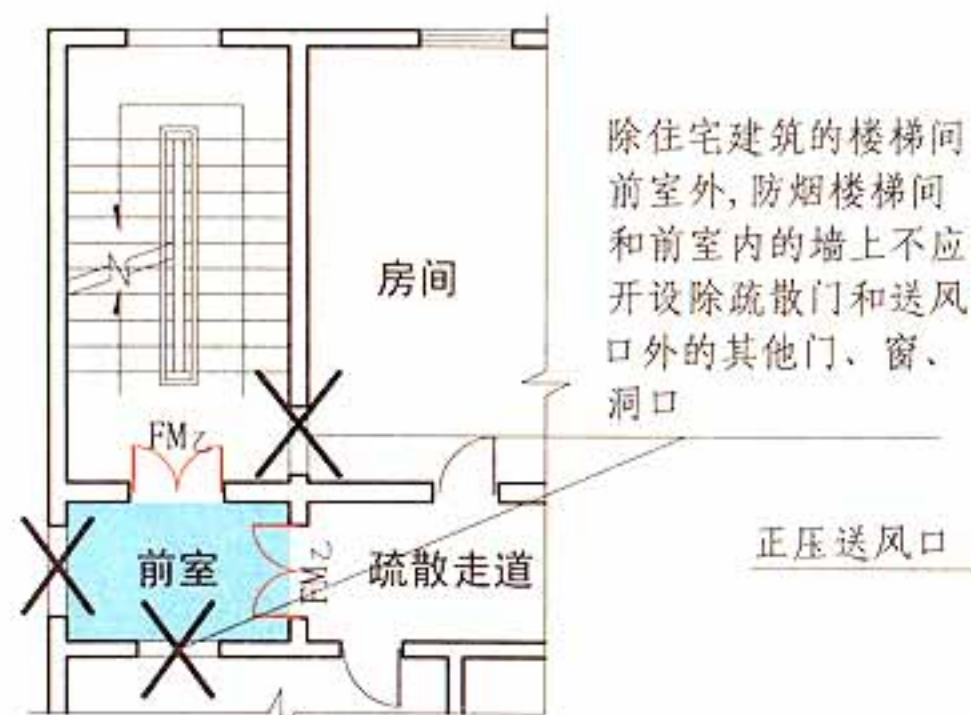
能自然通风且自然通风能满足要求的防烟楼梯间
