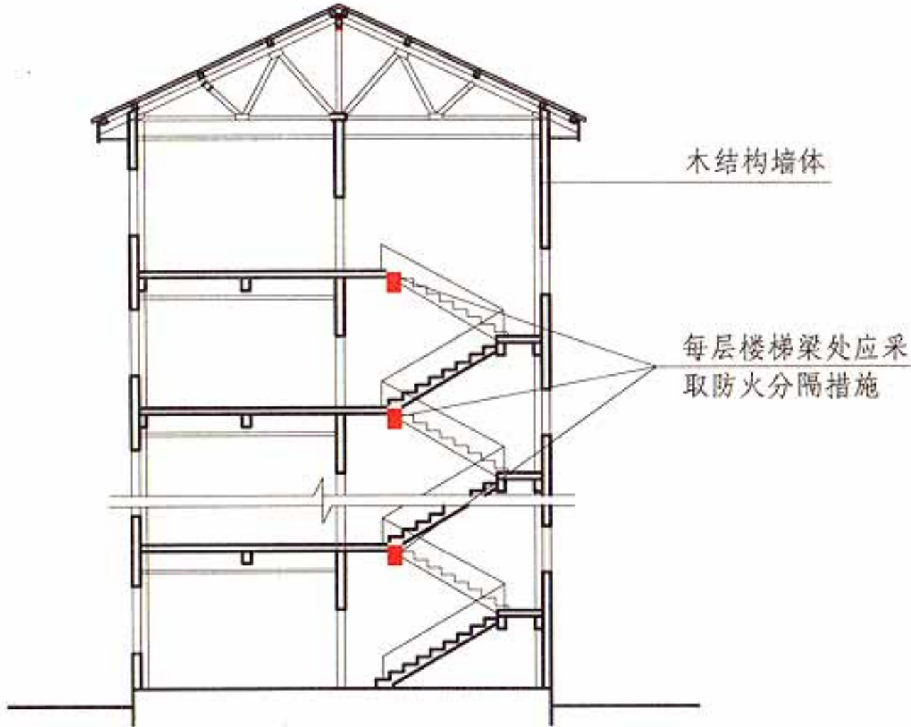
轻型木结构建筑剖面示意图
