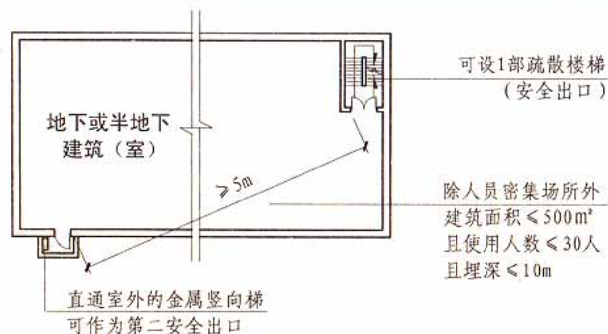
地下或半地下建筑(室)平面示意图
