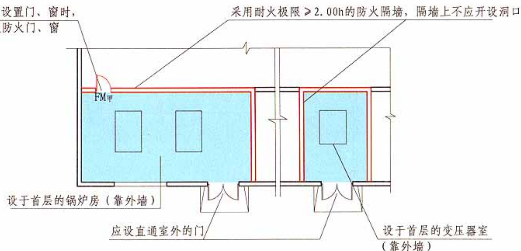
锅炉房、变压器室确需布置在民用建筑内首层时 平面示意图
