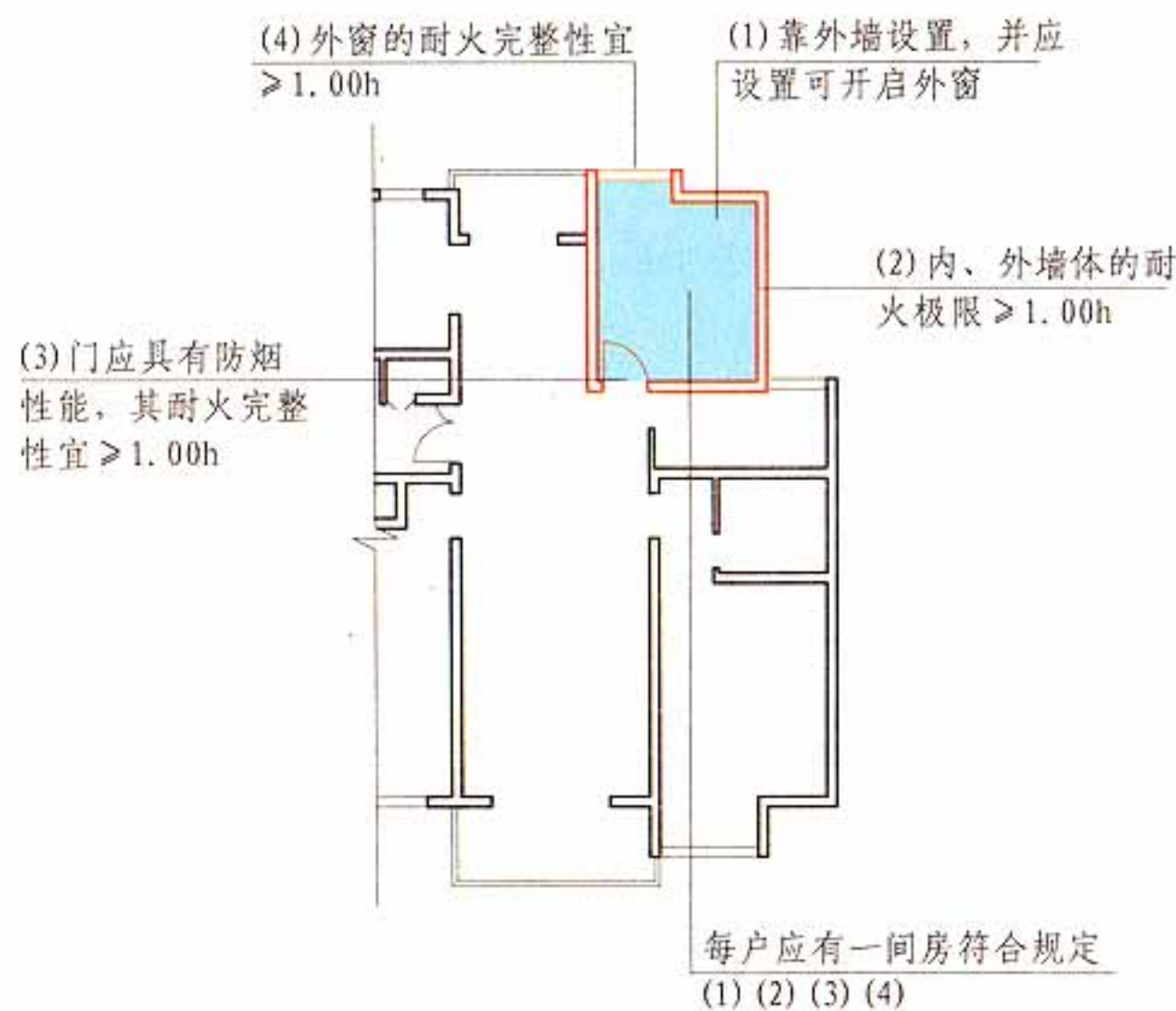
建筑高度 > 54m 的住宅建筑 平面示意图
