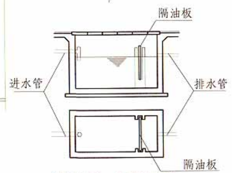
隔油池平、剖面示意图 (供参考)
