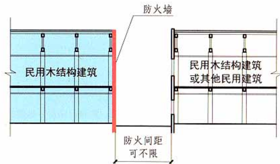
剖面示意图 11.0.10 图示5
