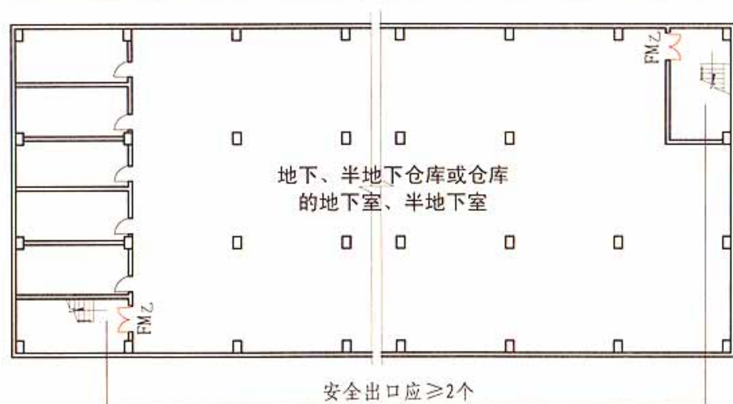
平面示意图
