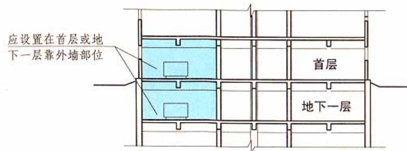
燃油或燃气锅炉房、变压器室确需设置在民用建筑内时 剖面示意图
