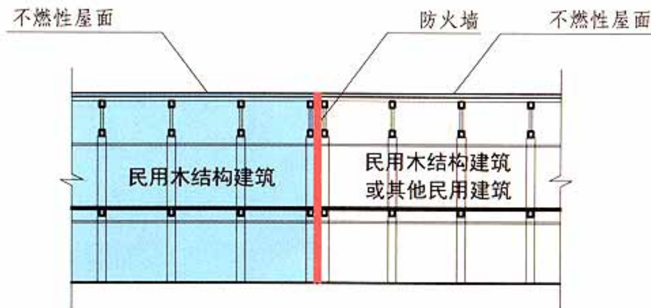
剖面示意图
