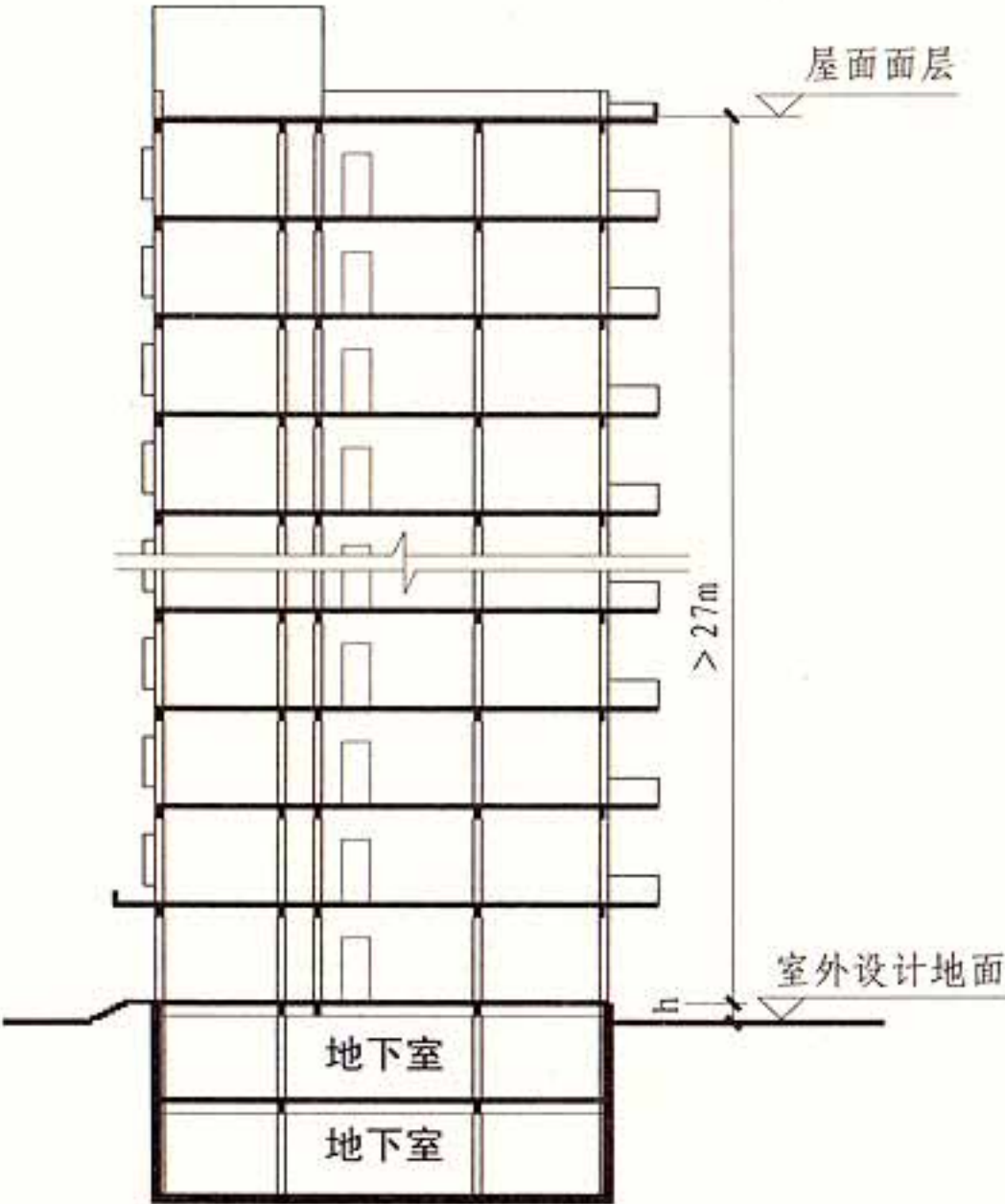
高层住宅建筑剖面示意图
