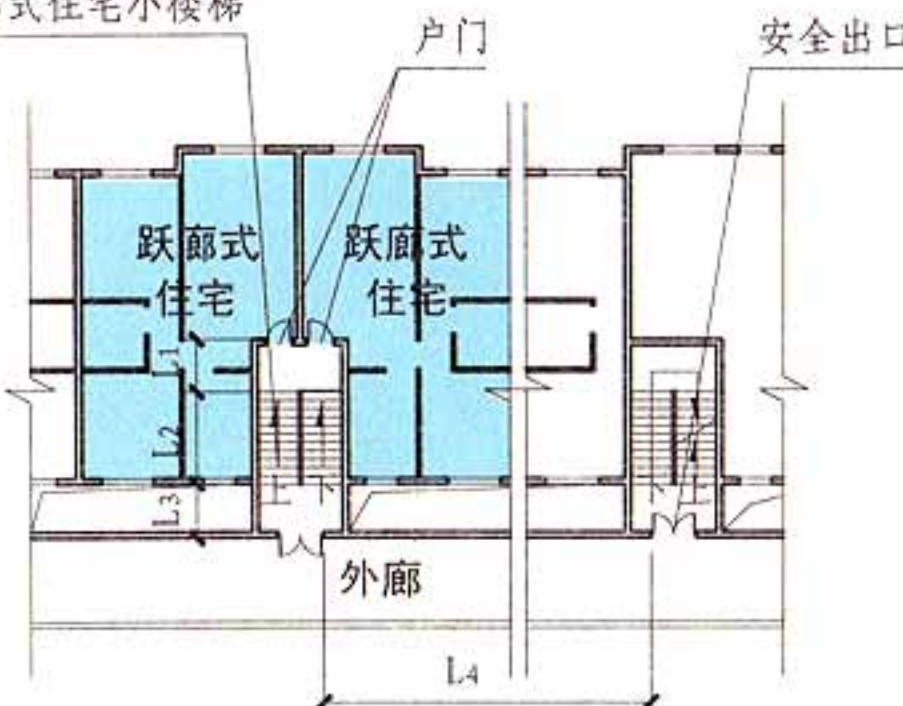
跃廊式住宅小楼梯
