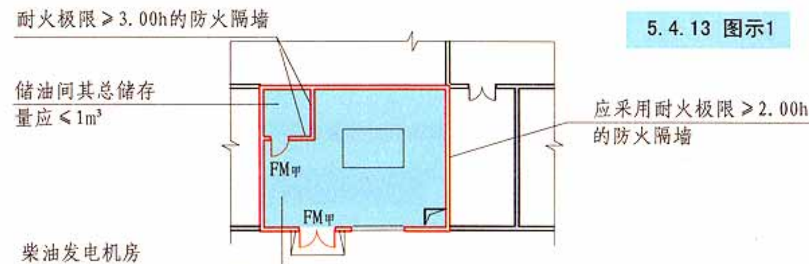
布置在民用建筑内的柴油发电机房 平面示意图
