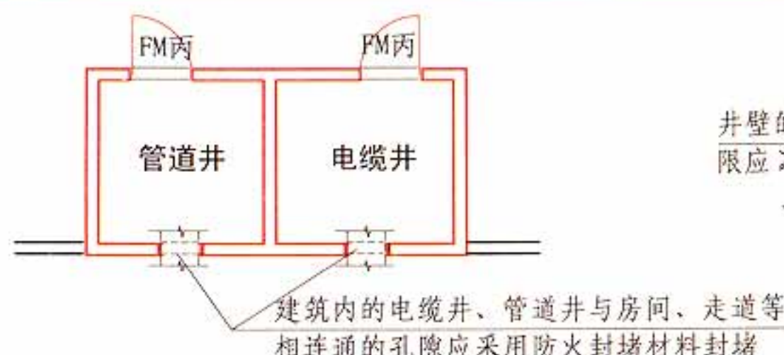
平面示意图 6.2.9 图示4
