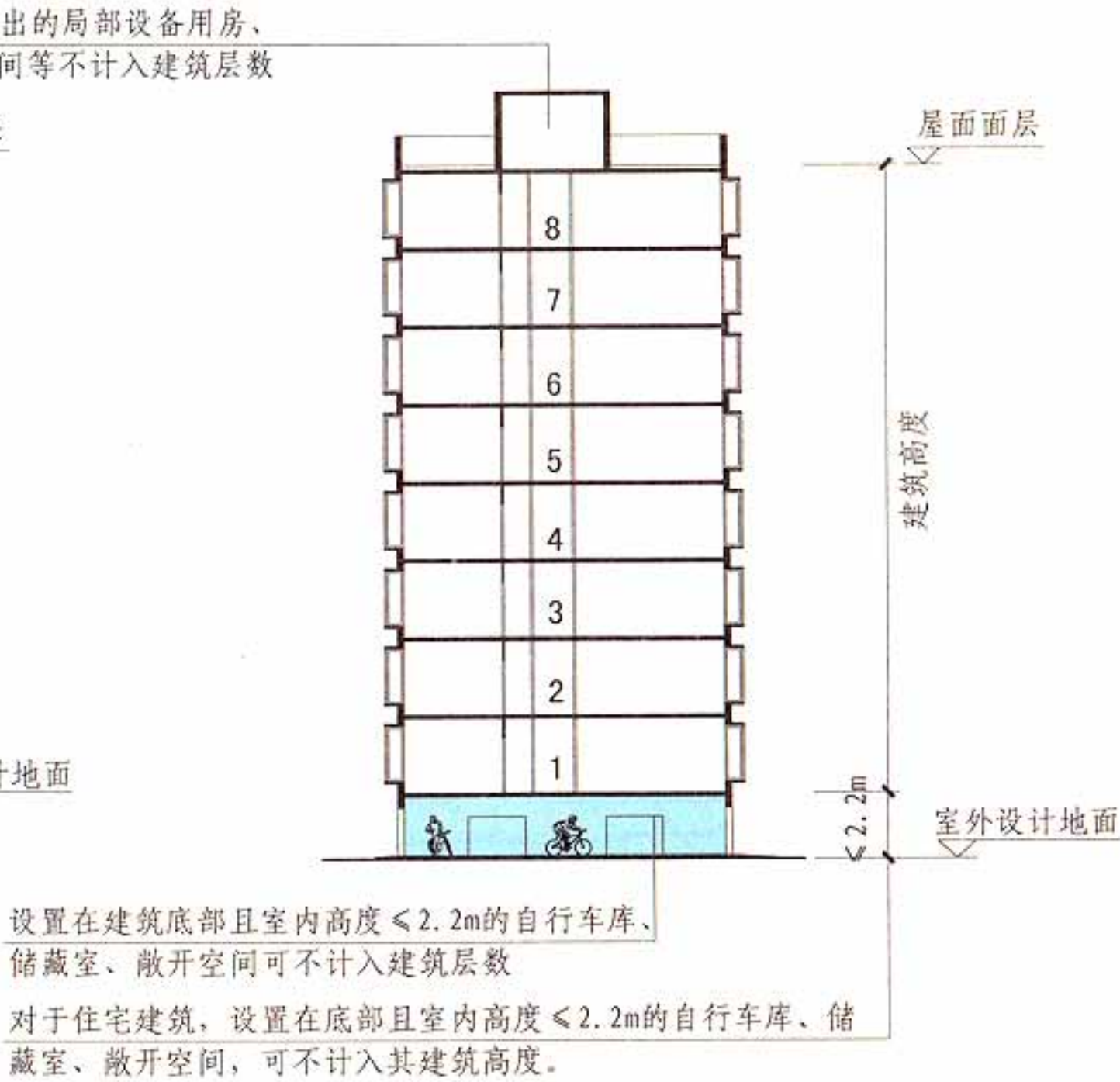
剖面示意图
