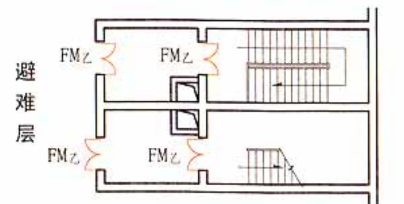
防烟楼梯在避难层同层错位平面示意图
