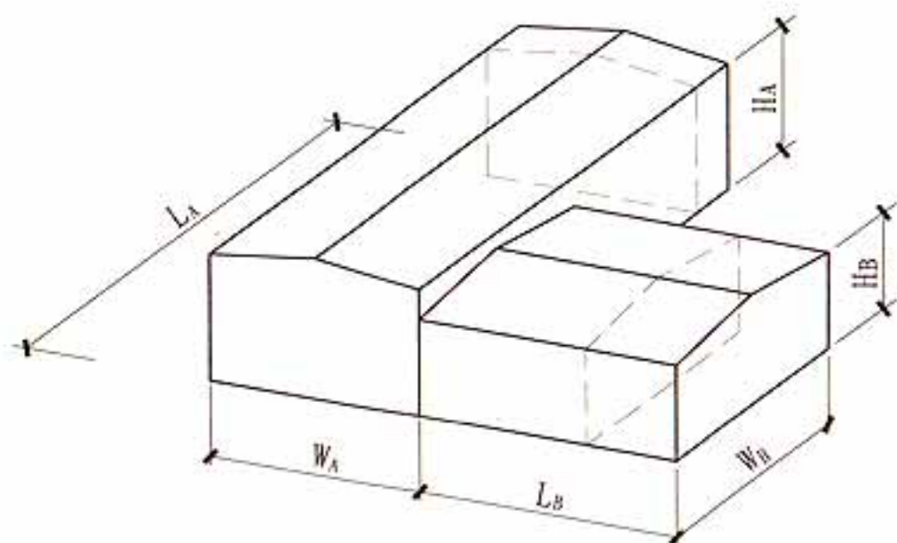
示意图
