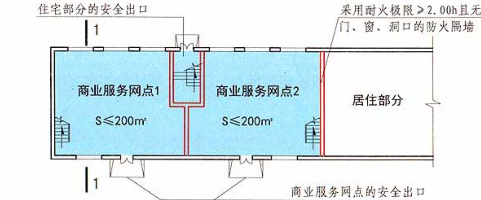
平面示意图
