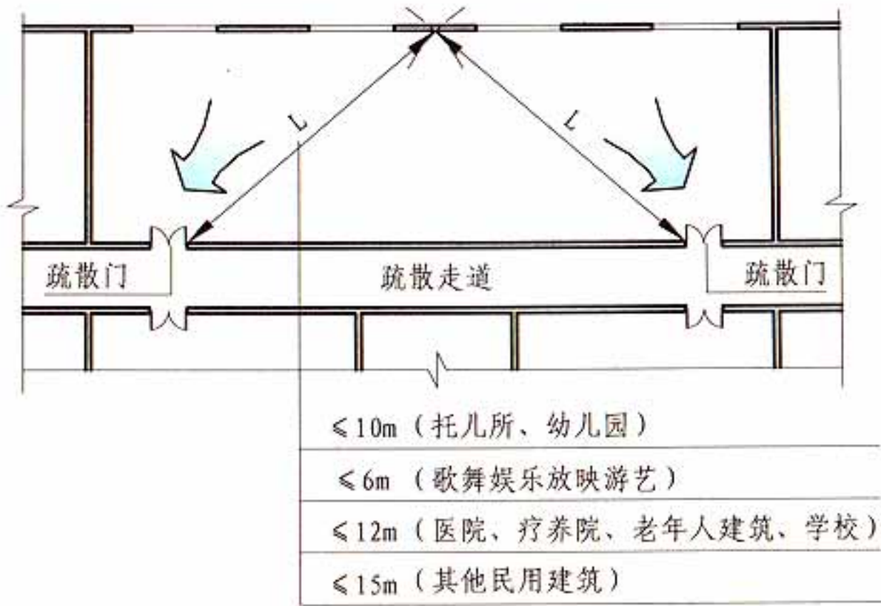
平面示意图
