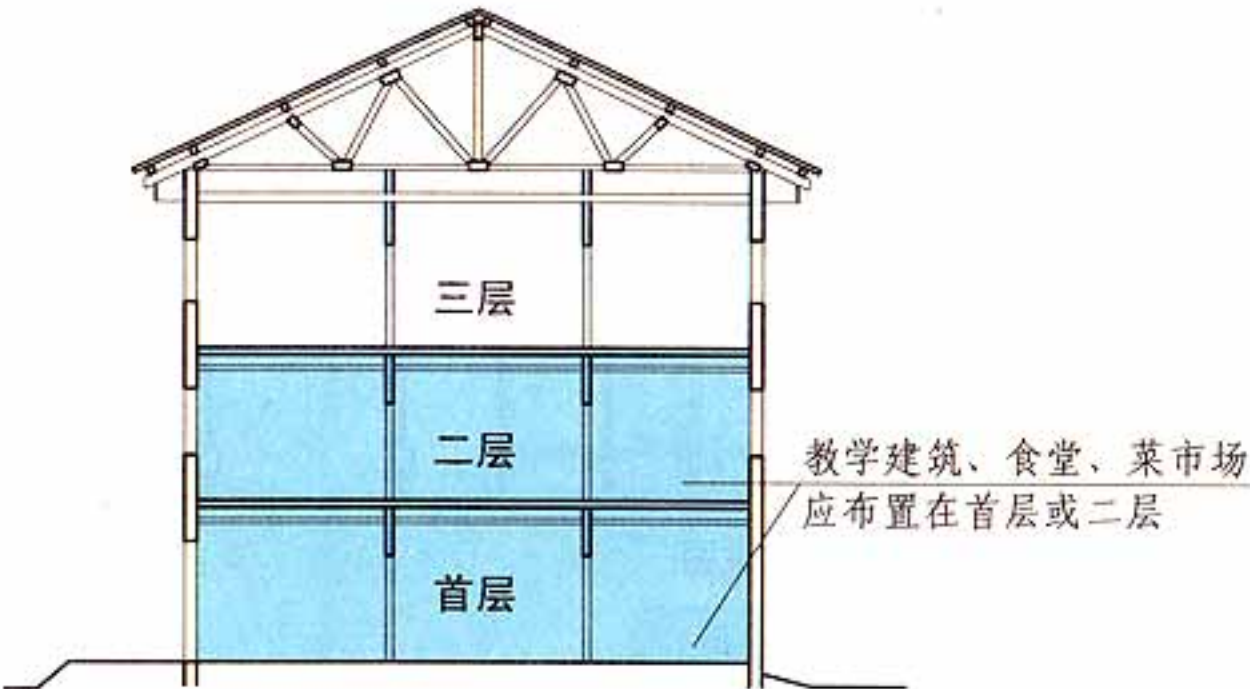
三级耐火等级建筑剖面示意图
