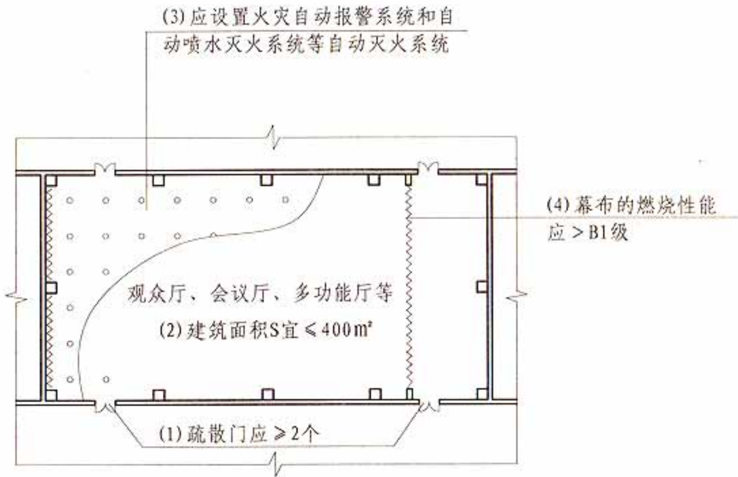
平面示意图
