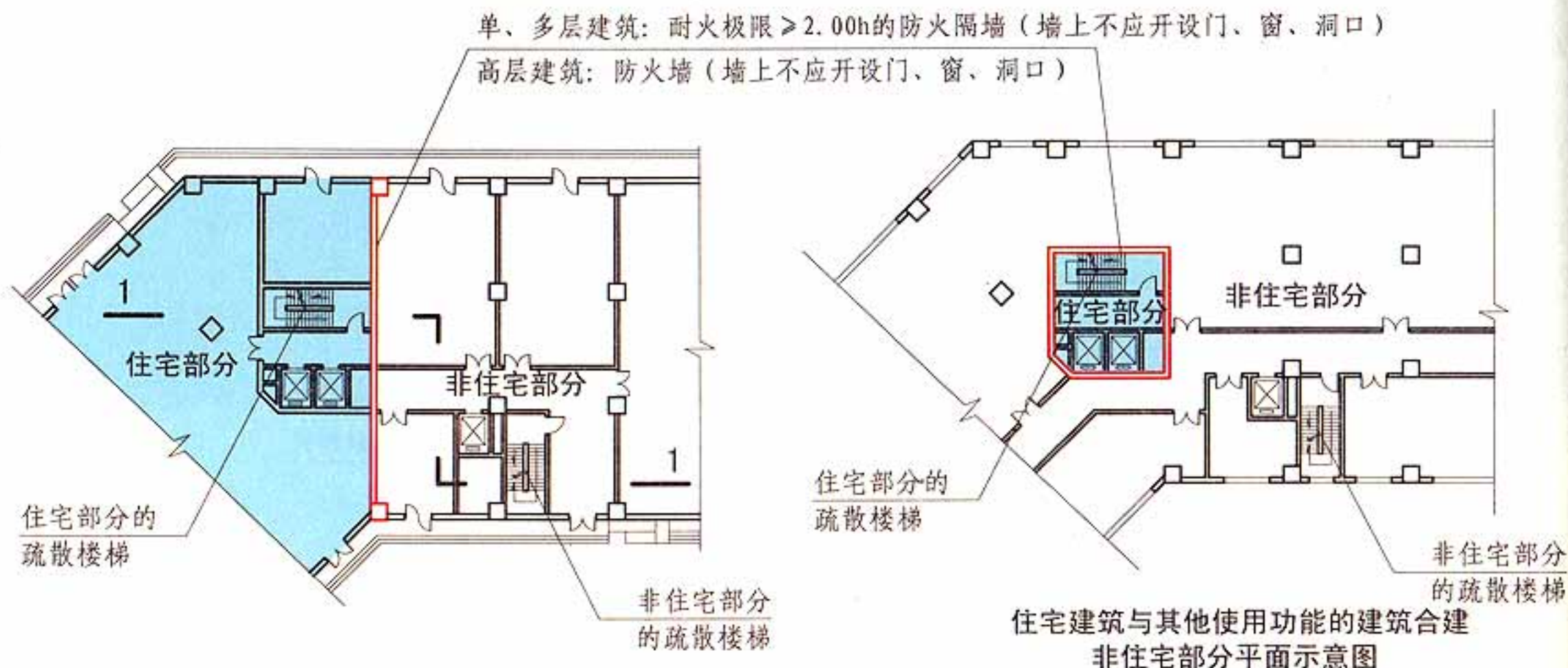
住宅建筑与其他使用功能的建筑合建 首层平面示意图
