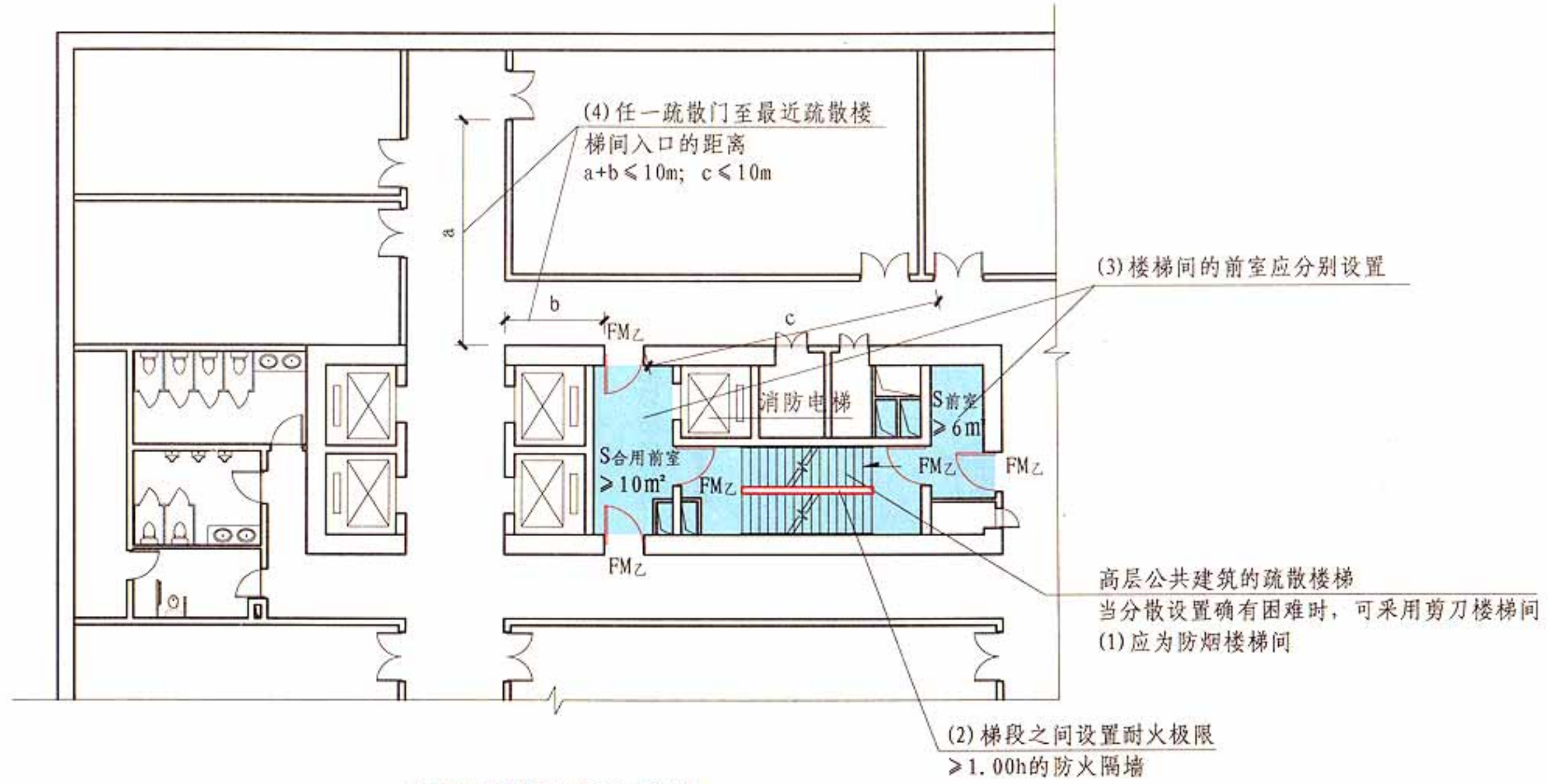
高层公共建筑 平面示意图
