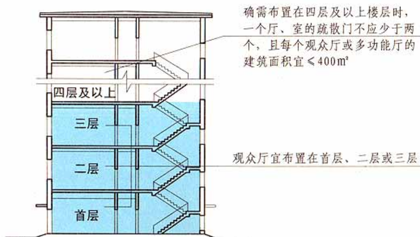
一、二级耐火等级多层建筑 剖面示意图
