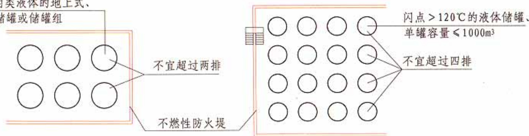
平面示意图
