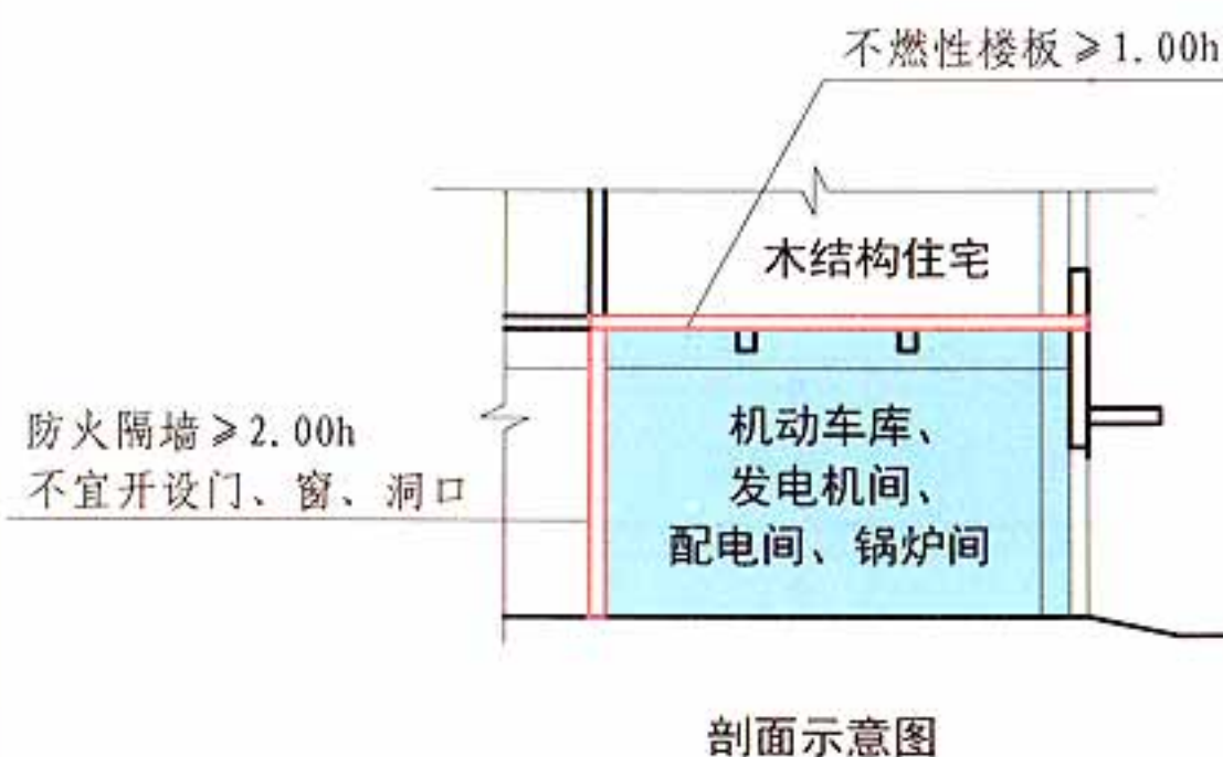
木结构住宅
