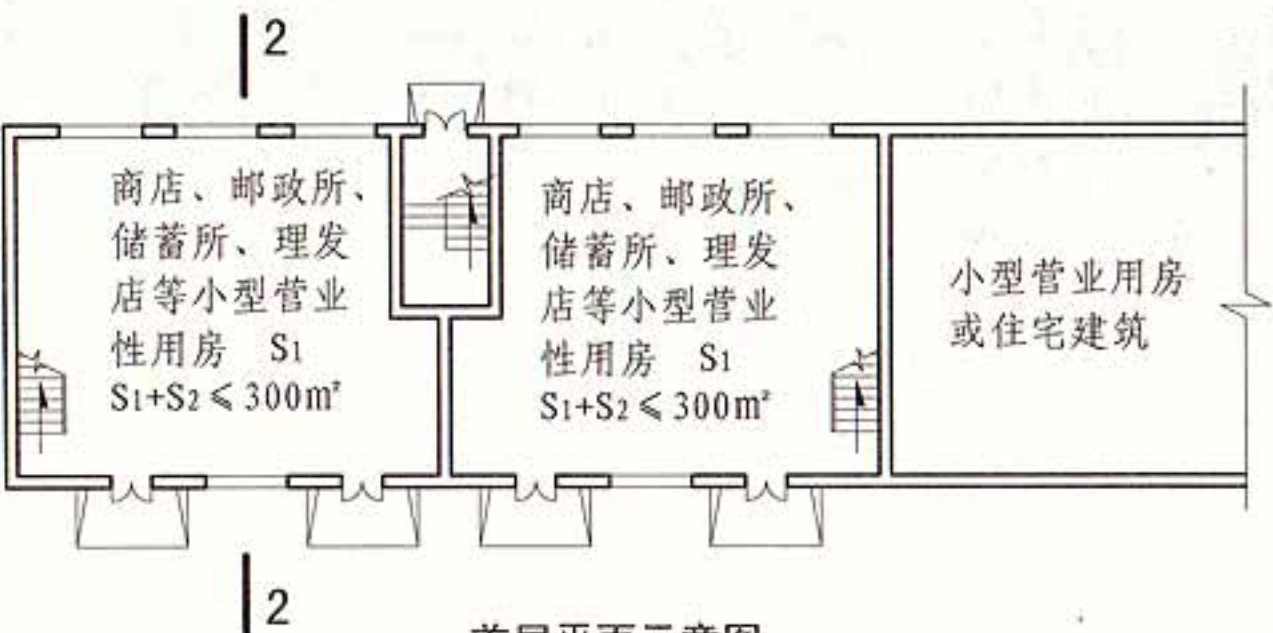
首层平面示意图
