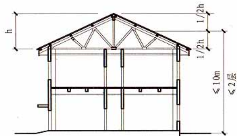
普通木结构建筑
