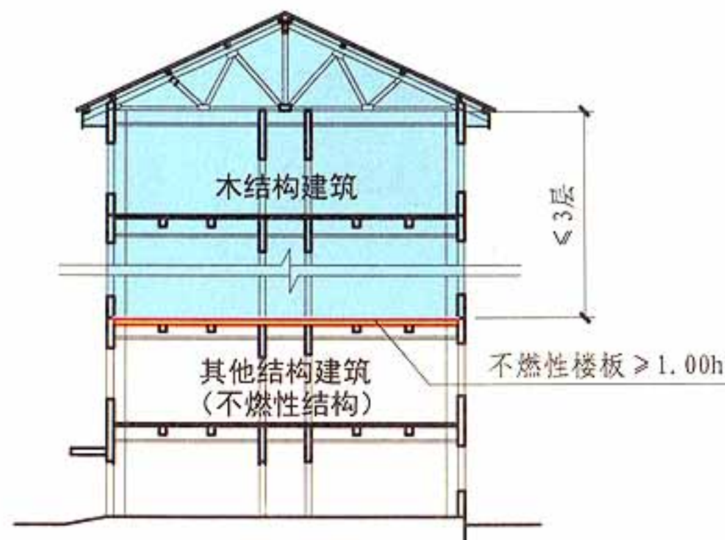
剖面示意图
