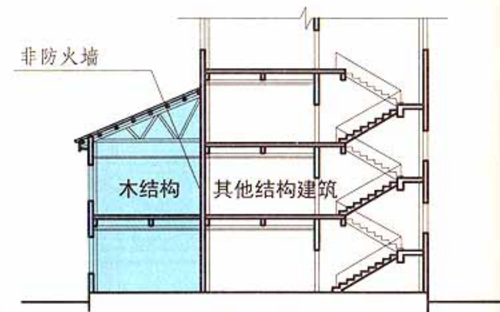
剖面示意图
