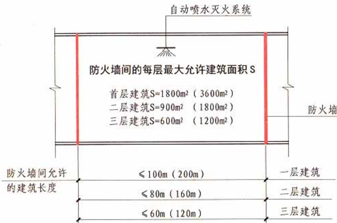
平面示意图
