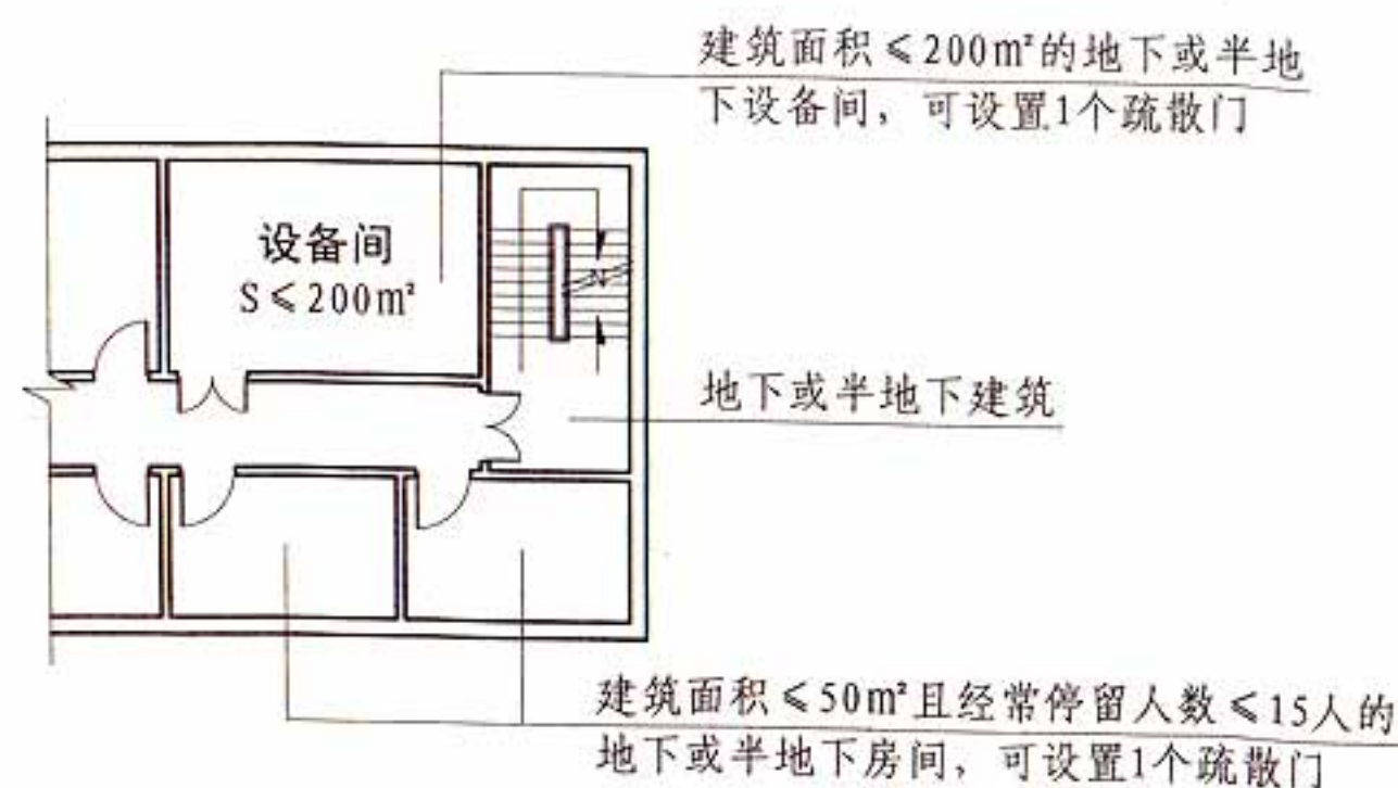
地下或半地下建筑(室)平面示意图
