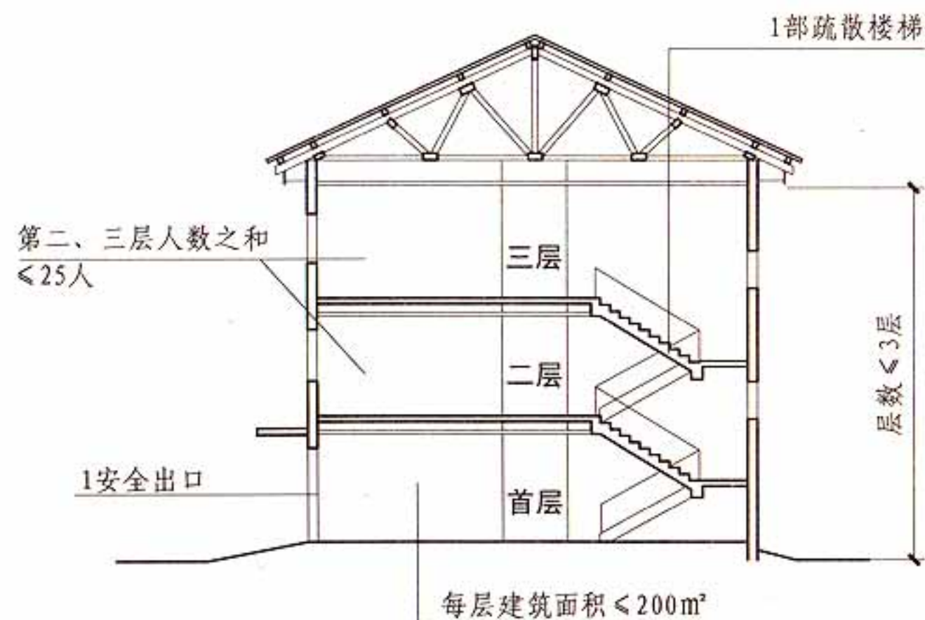
2-2 (三级耐火等级建筑)
