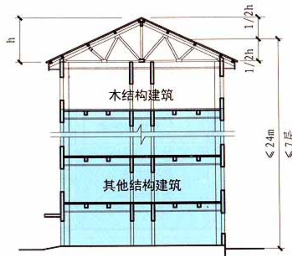
木结构组合建筑
