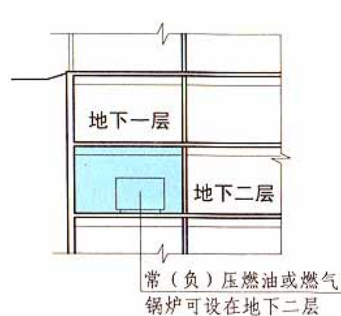
剖面示意图
