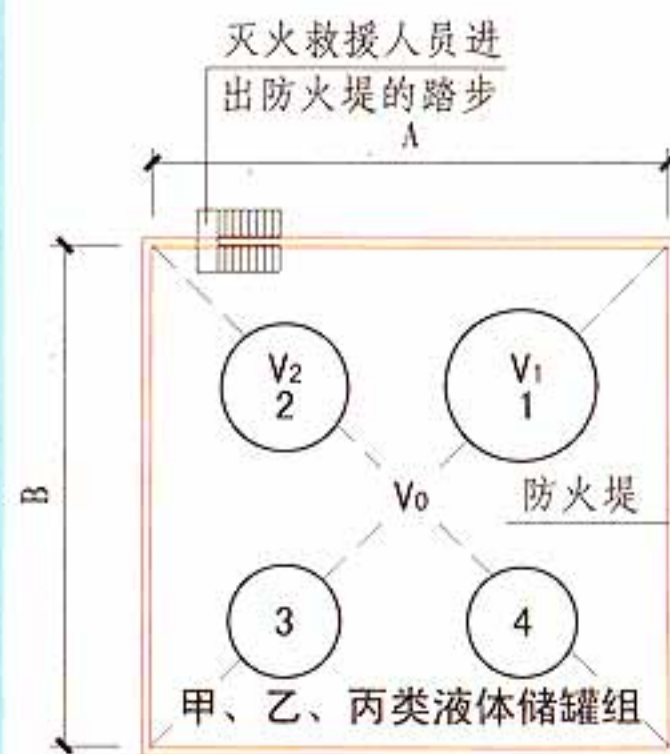
平面示意图
