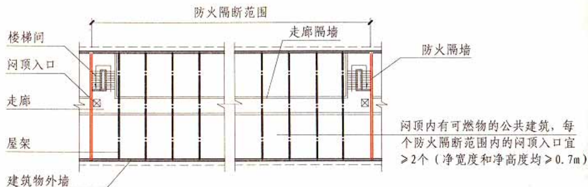
公共建筑闷顶平面示意图
