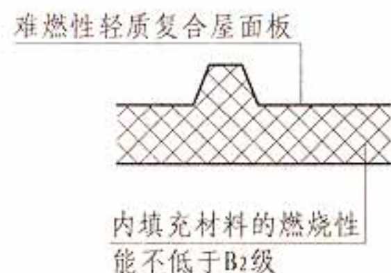
一、二级耐火等级 丁、戊类厂房（仓库） 屋面板材料
