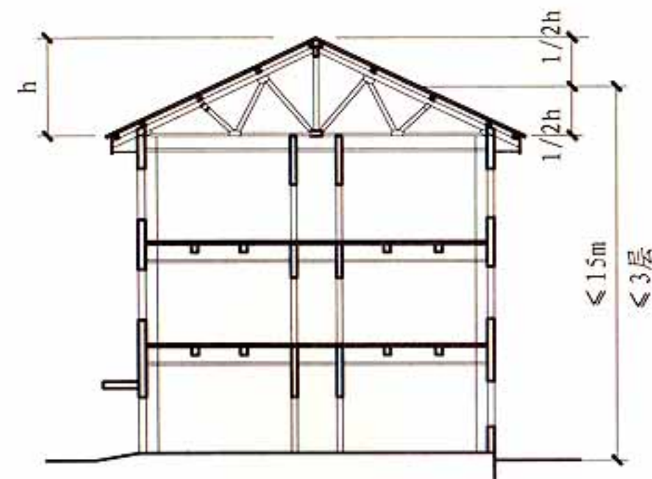
胶合木结构建筑
