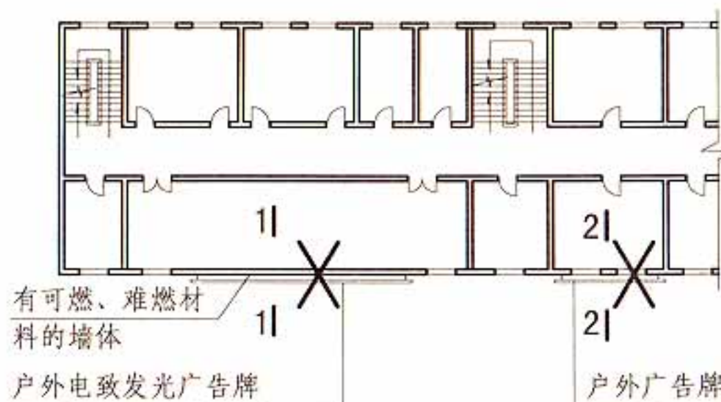
平面示意图
