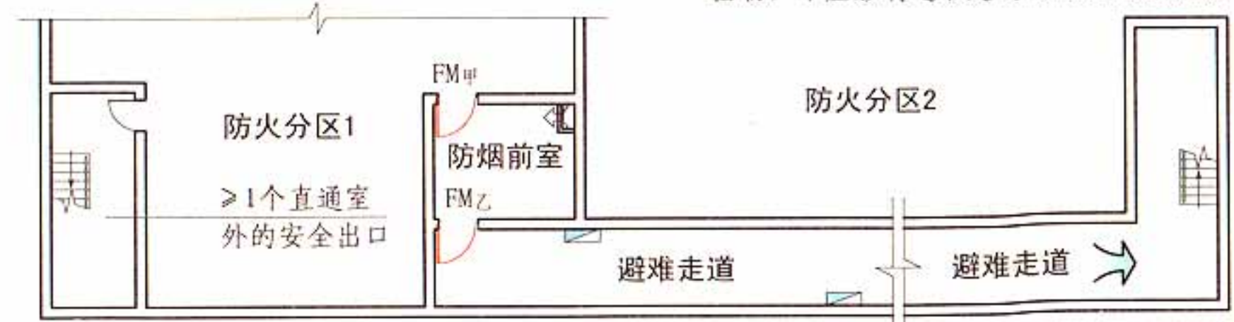
6.4.14 图示2 仅与一个防火分区相连通的避难走道示意图
