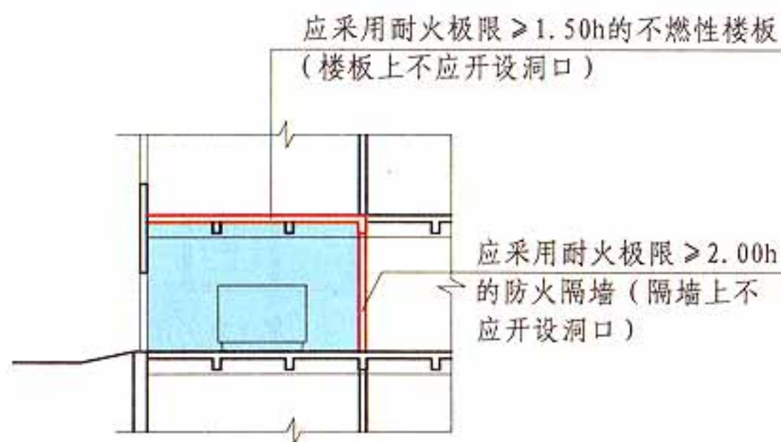
锅炉房、变压器室确需布置在民用建筑内时 剖面示意图
