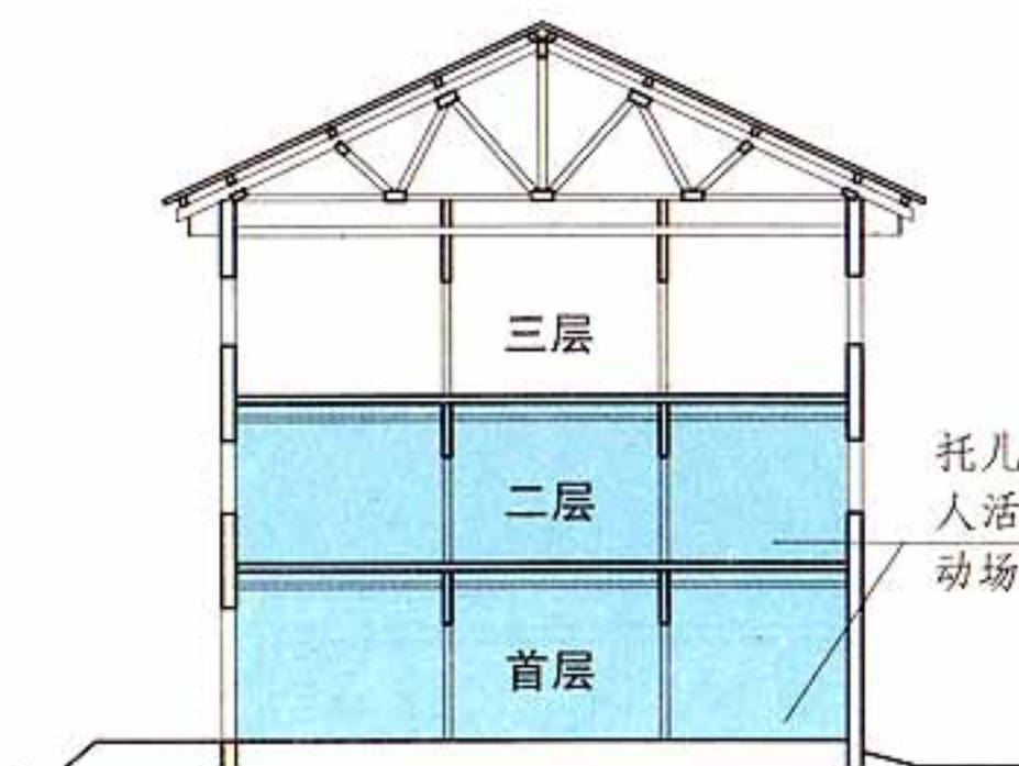
剖面示意图 三级耐火等级建筑
