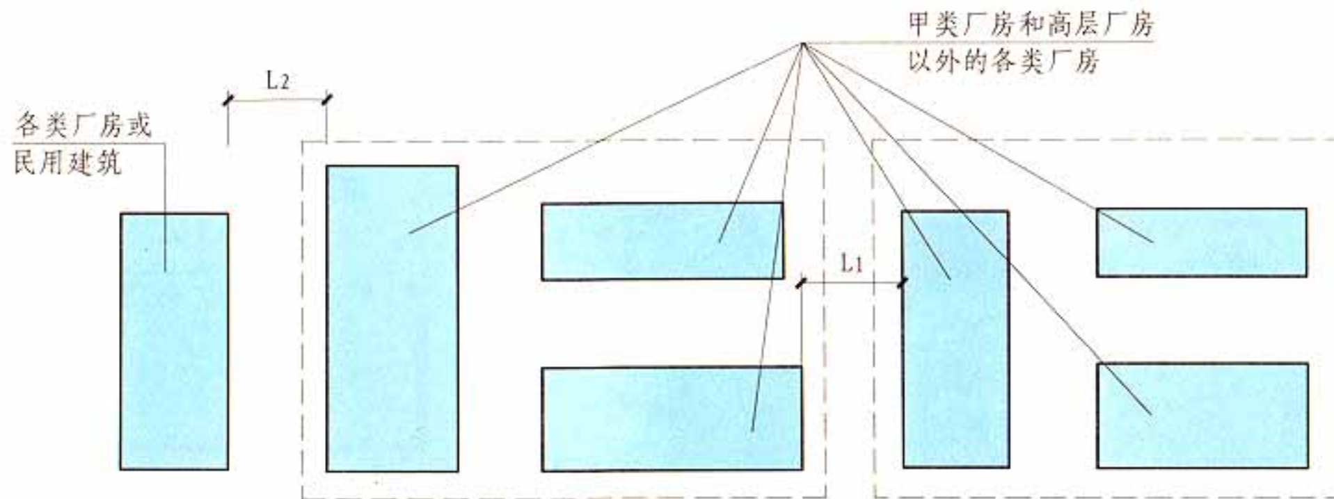
组与组或组与相邻建筑的防火间距平面布置示意图
