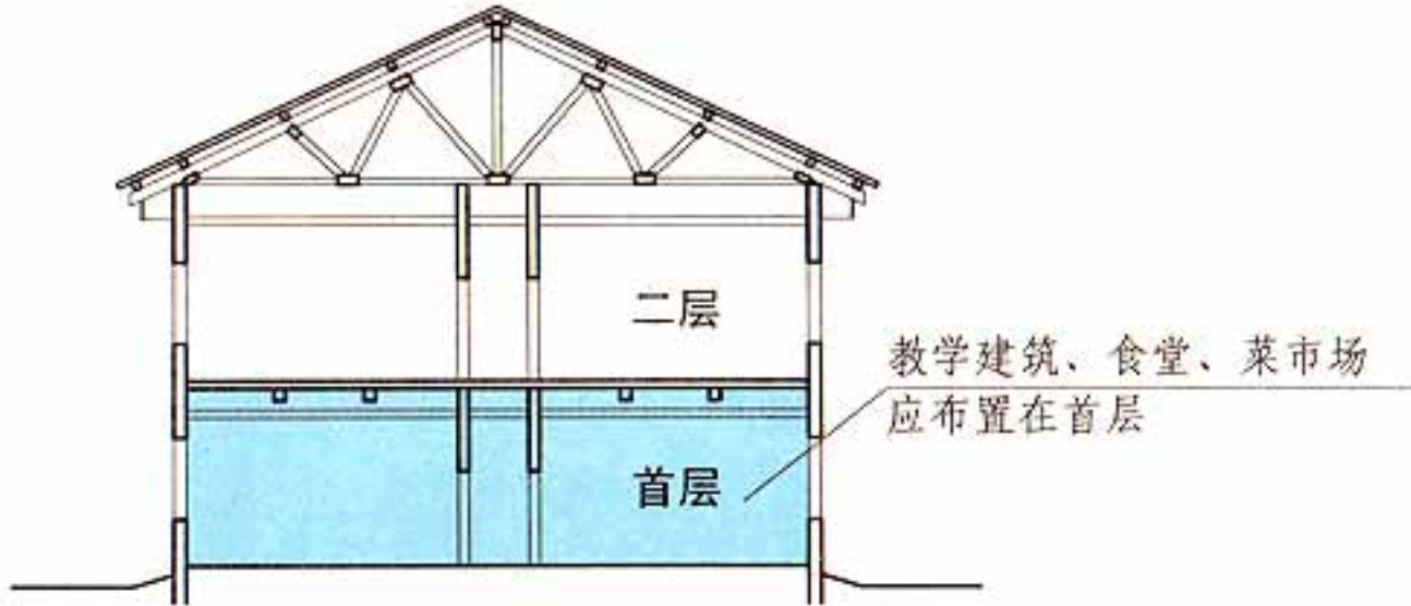
四级耐火等级建筑剖面示意图
