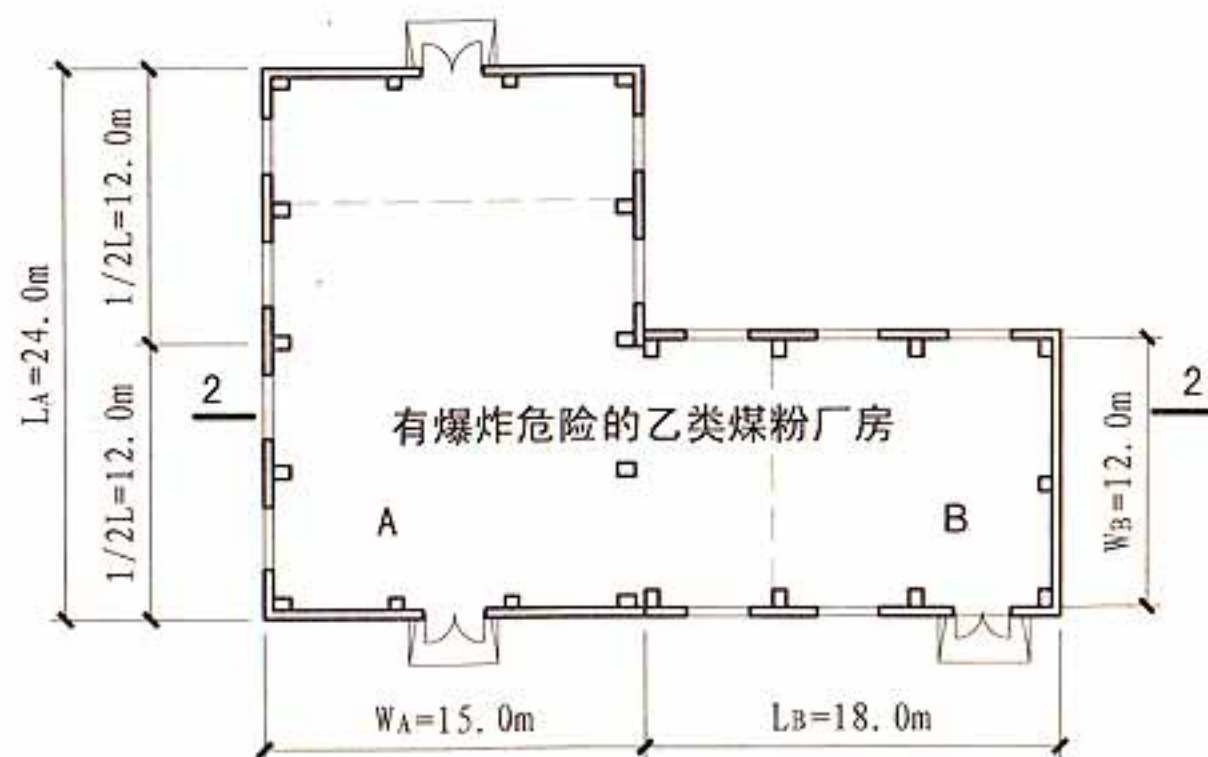
平面图
