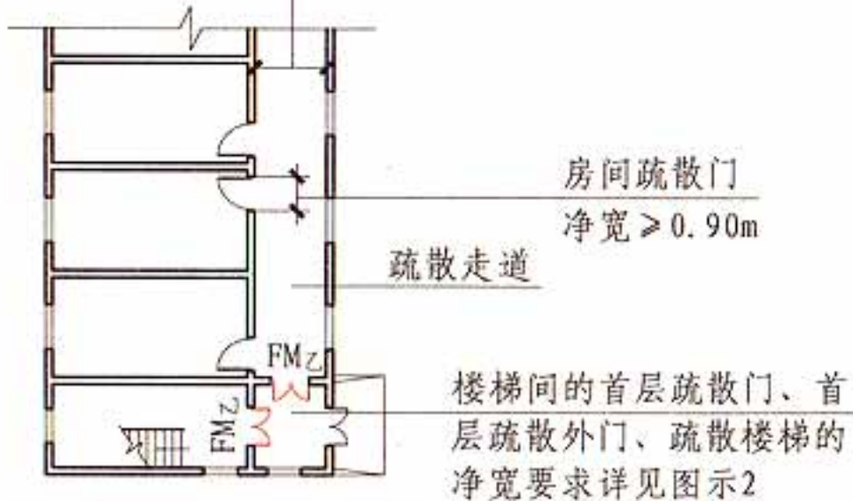
高层公共建筑 平面示意图 5.5.18 图示3
