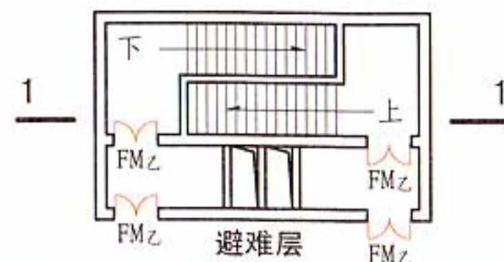
防烟楼梯在避难层上下层断开平面示意图
