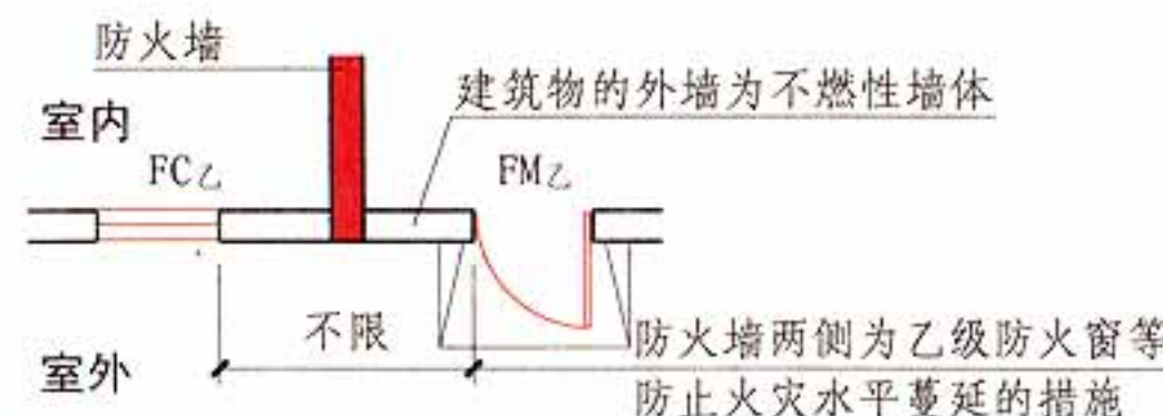
平面示意图
