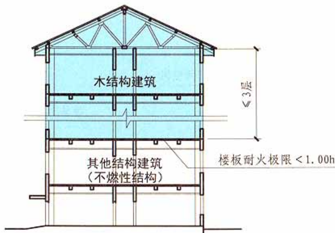
剖面示意图
