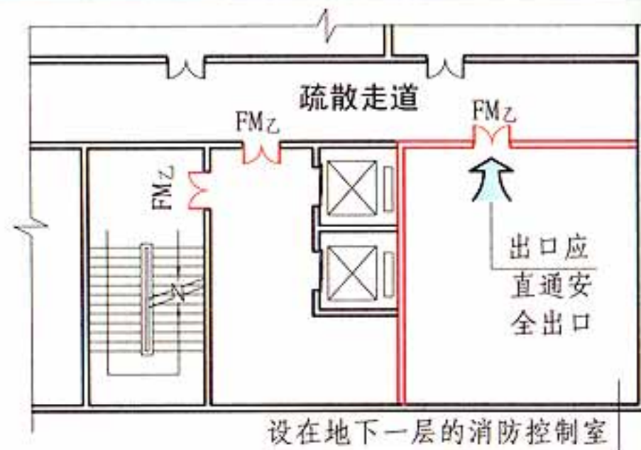
地下一层平面示意图
