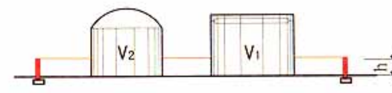
固定顶储罐与浮顶储罐同组布置 V_0 \geq V_2 与 V_0 \geq 0.5V_1 取两者中的较大值 V_1 为最大浮顶储罐的容量 V_2 为最大固定顶储罐的容量
