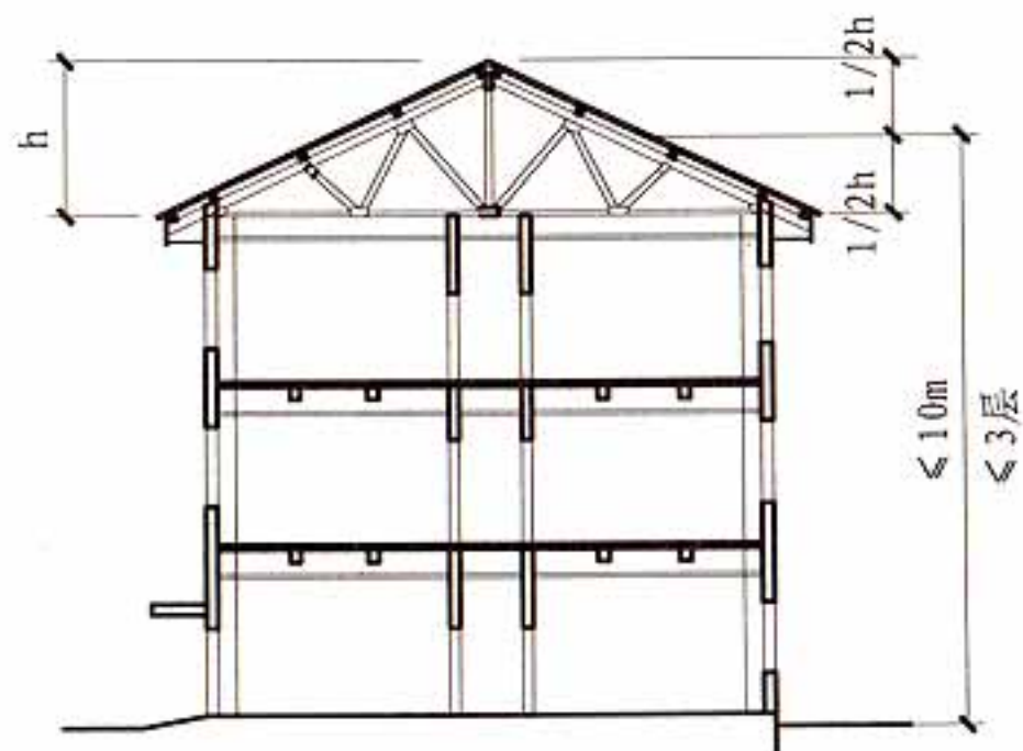
轻型木结构建筑
