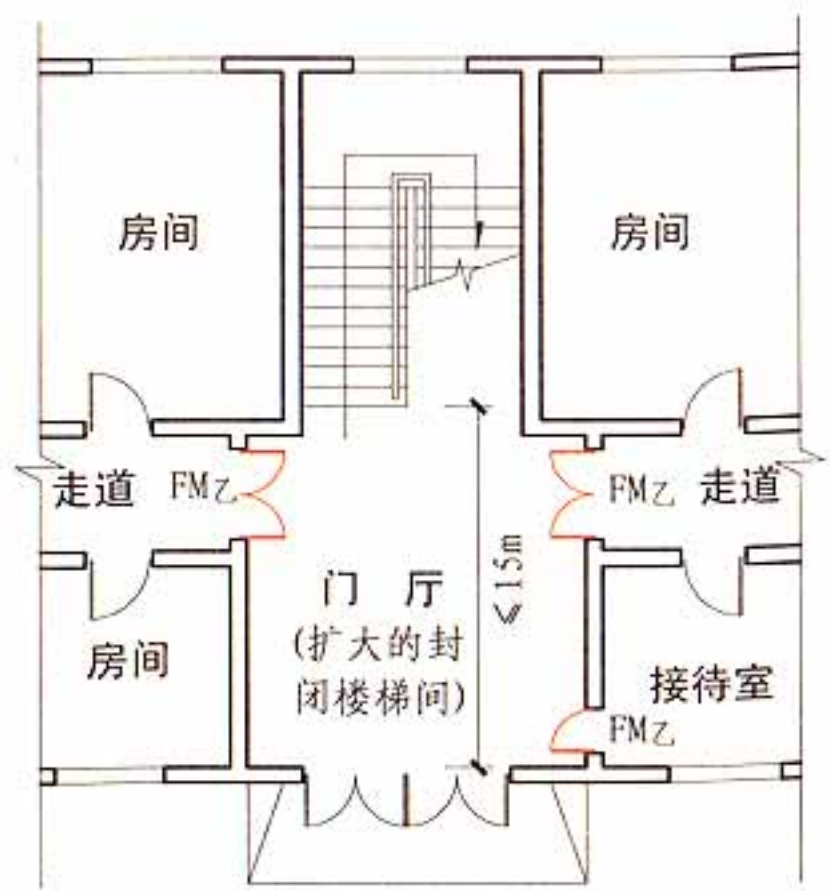
不能自然通风或自然通风不能满足要求的封闭楼梯间
