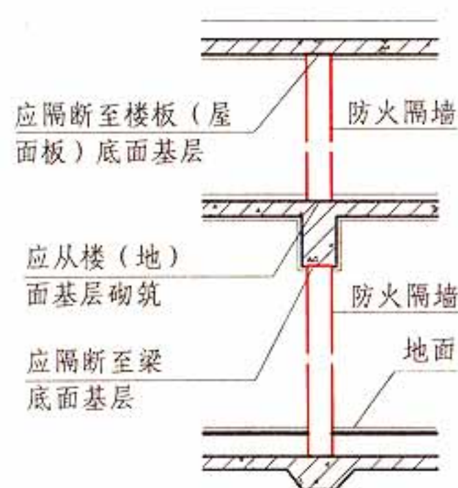
剖面示意图
