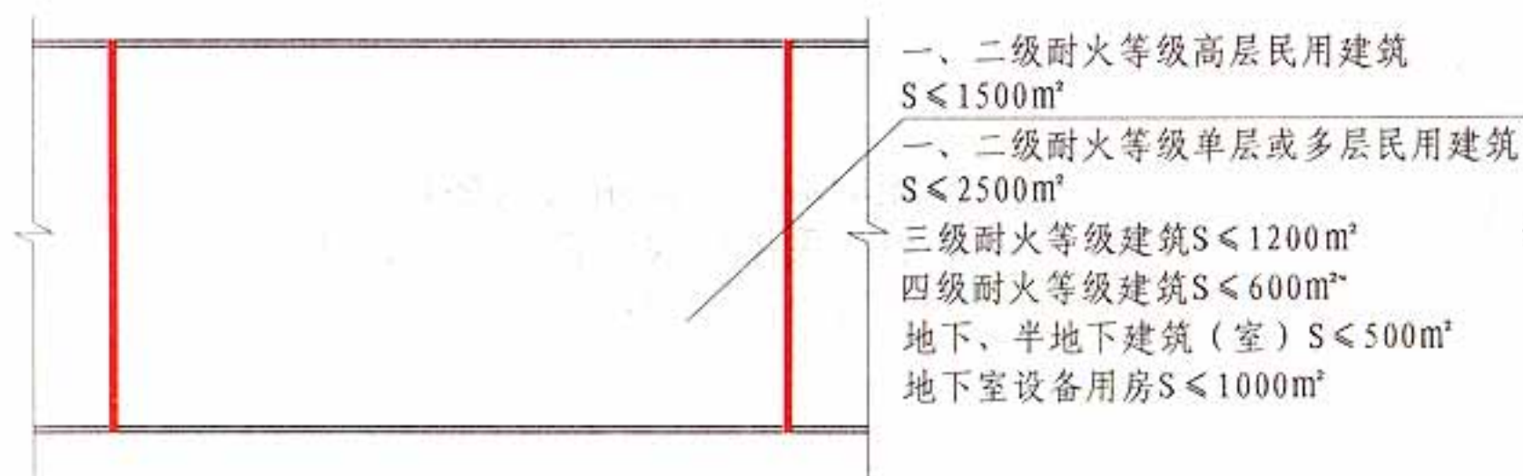
防火分区的最大允许建筑面积S
