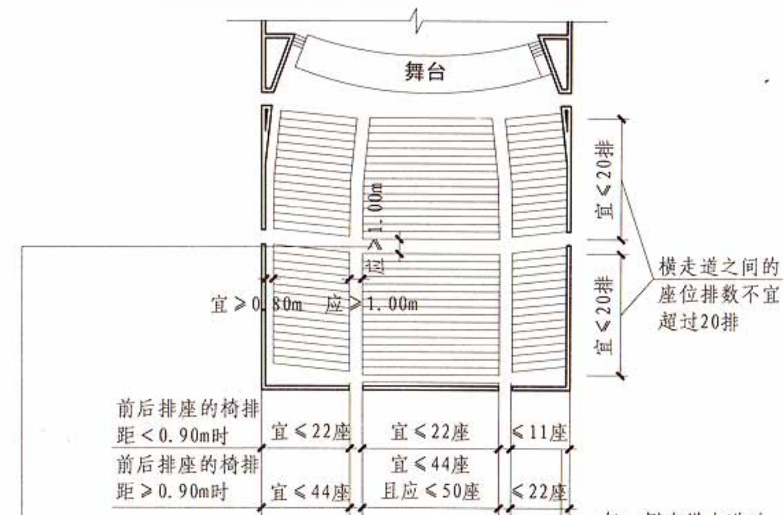
观众厅 (剧院、电影院、礼堂等) 平面示意图
