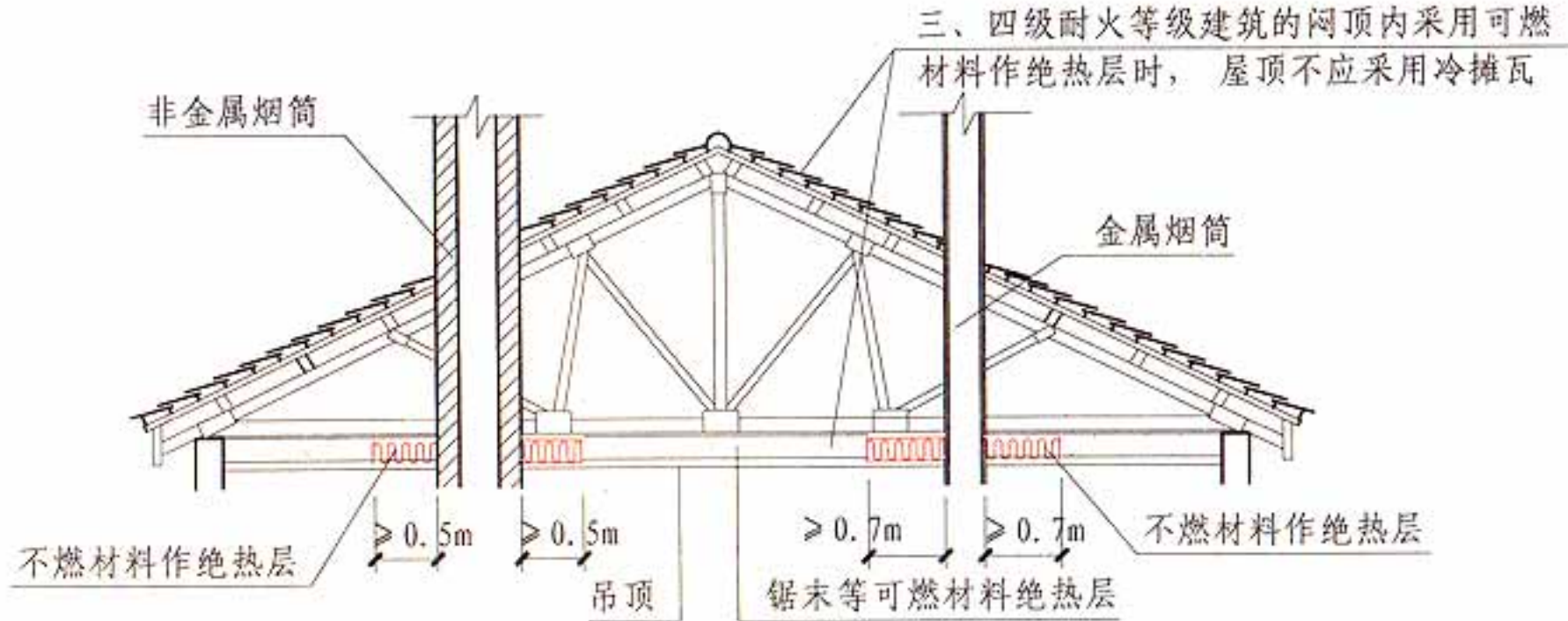
三、四级耐火等级建筑的闷顶
