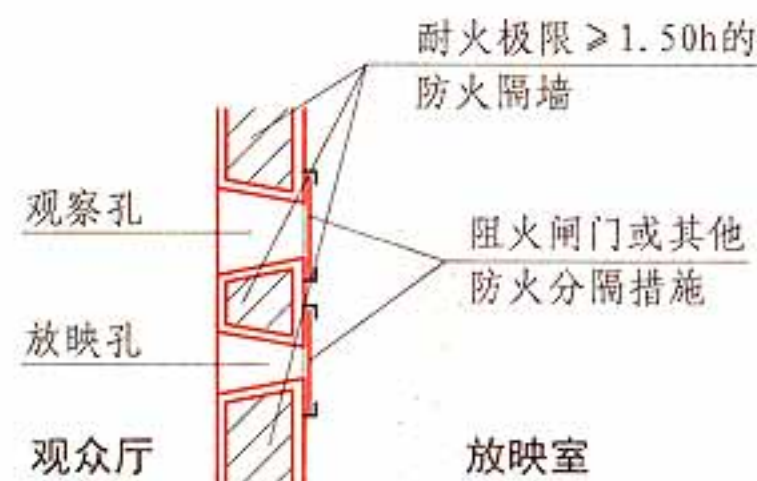
平面示意图
