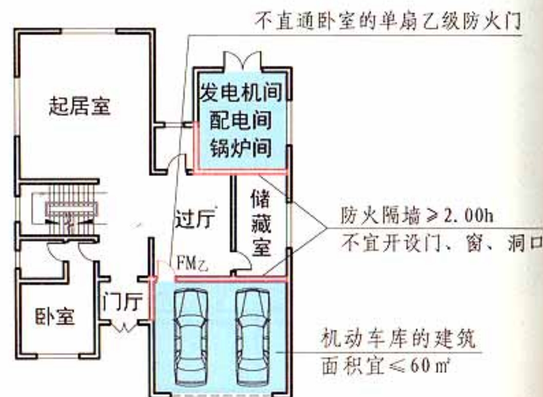
平面示意图
