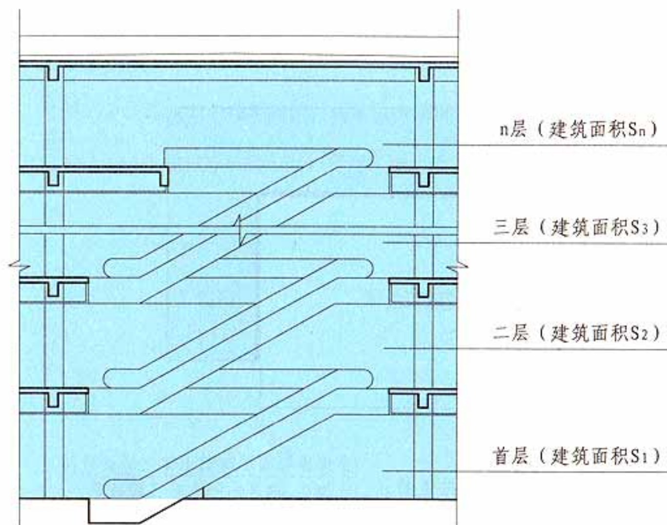
自动扶梯 剖面示意图
