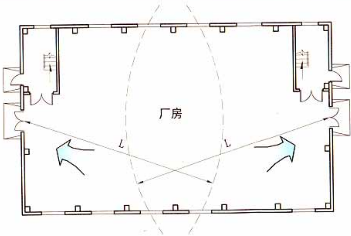
平面示意图
