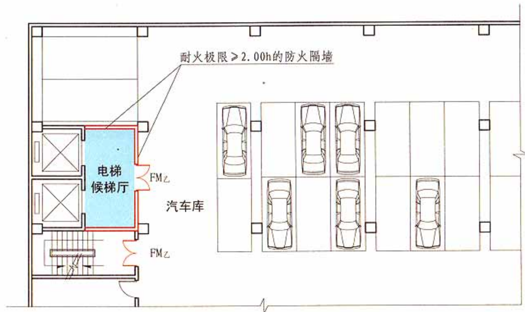
平面示意图
