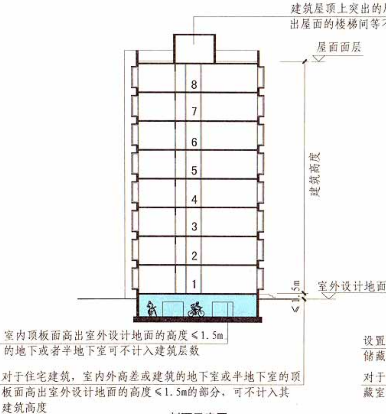
剖面示意图
