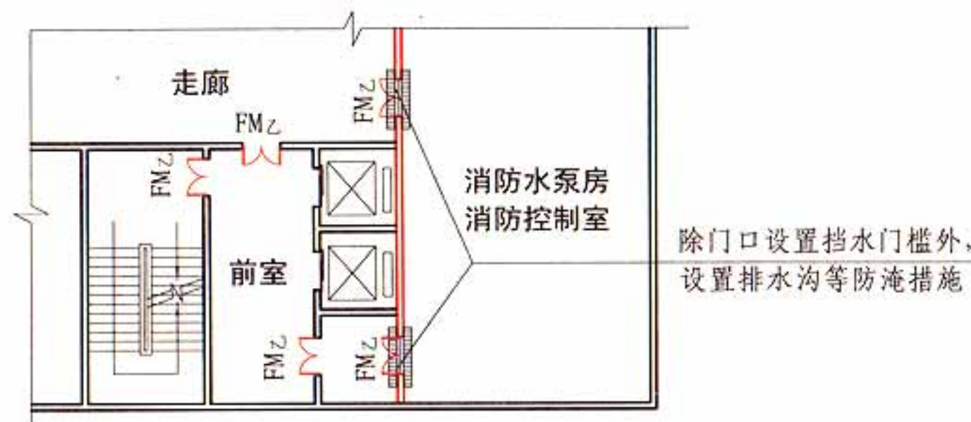
设在建筑地下的消防水泵房或消防控制室
