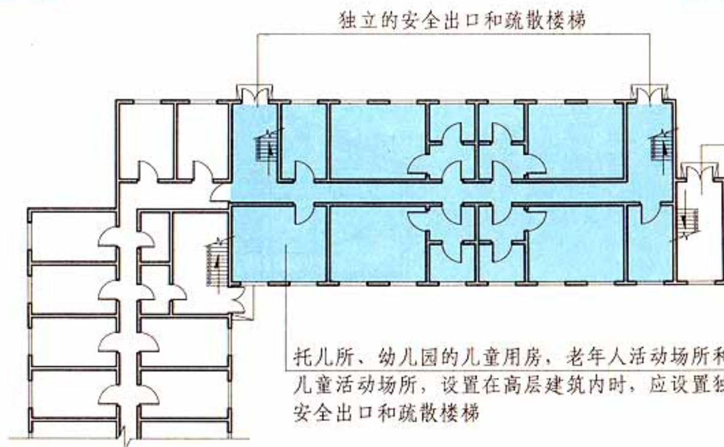
高层建筑平面示意图
