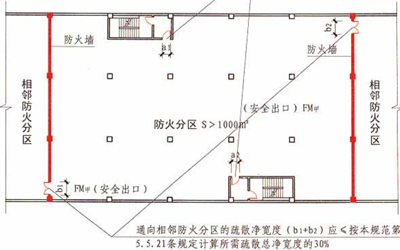
一、二级耐火等级公共建筑 平面示意图
