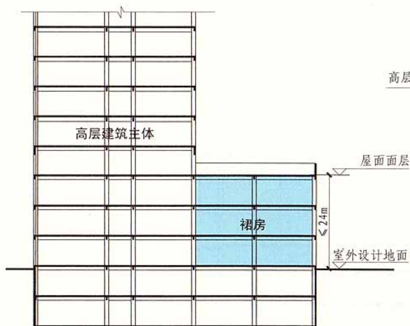
剖面示意图
