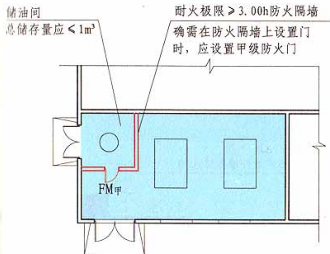
锅炉房内设置储油间时平面示意图
