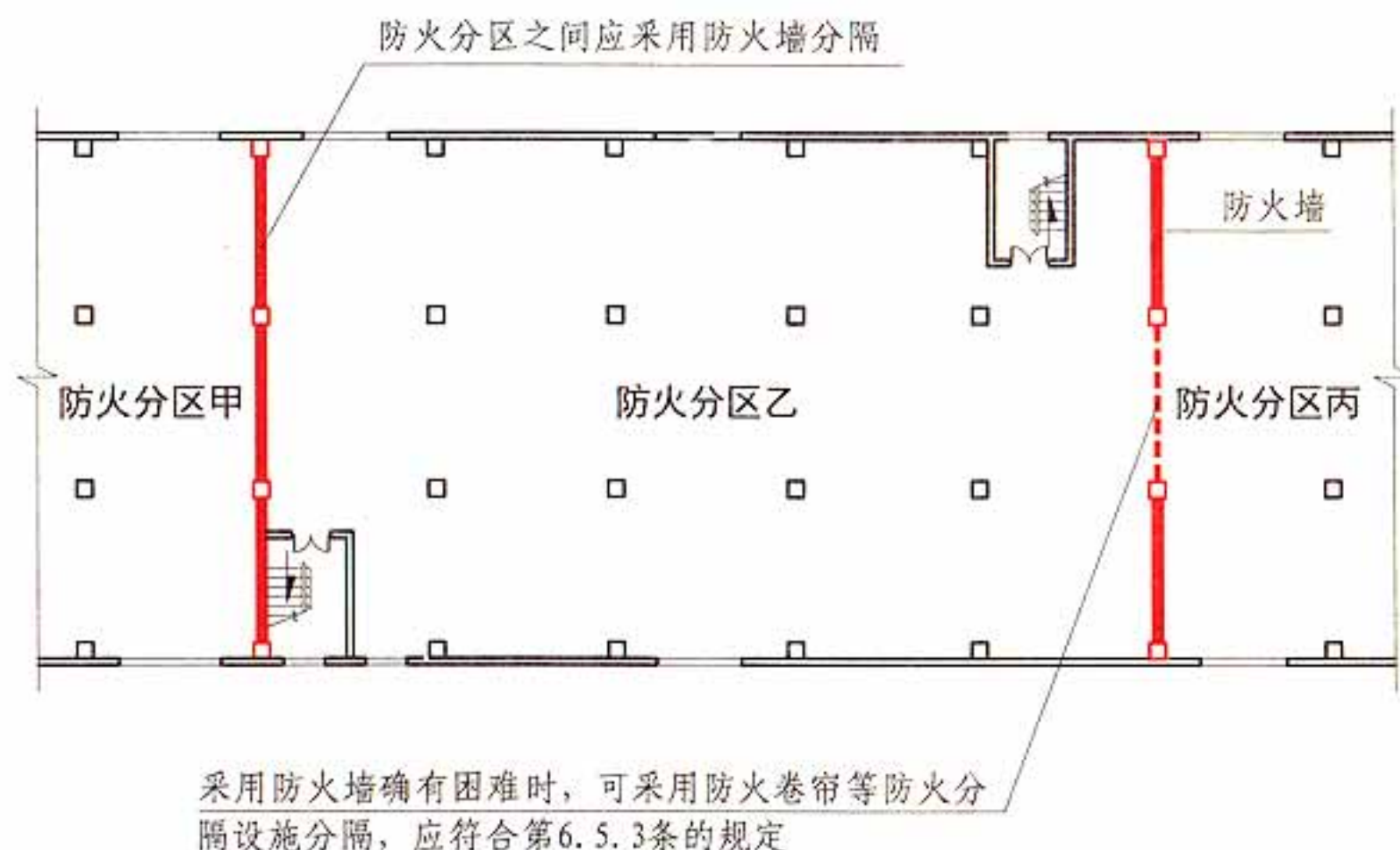
平面示意图
