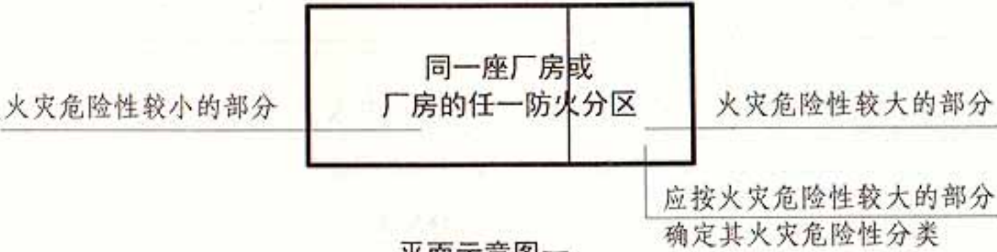
平面示意图一 3.1.2 图示1
